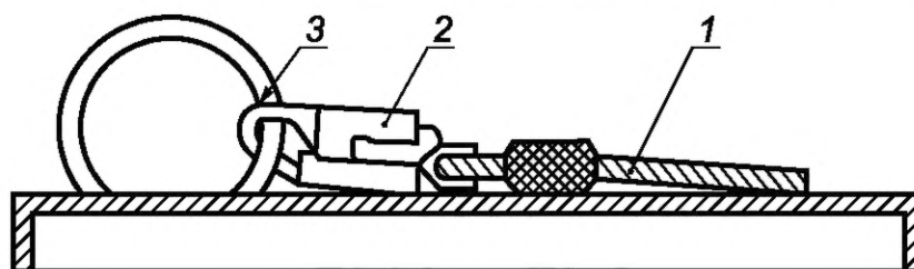
Рисунок 1 — Схемы установки страховочного каната выше плоскости опоры для ступней ног
