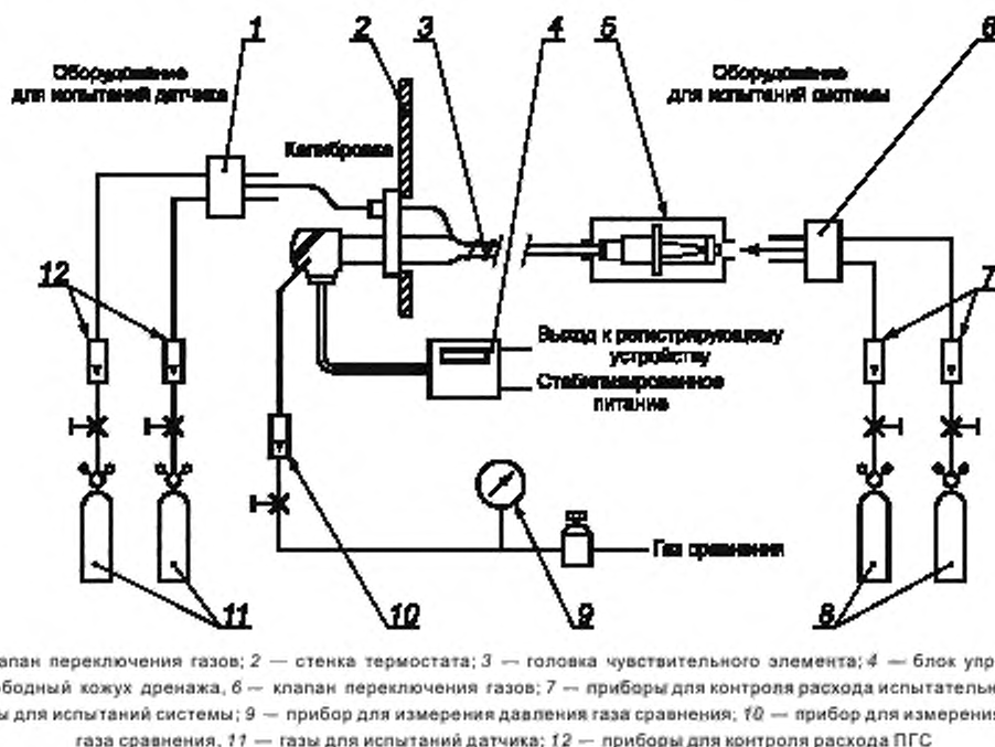
Рисунок 1 — Установка для определения динамических характеристик газоанализаторов «на месте»
