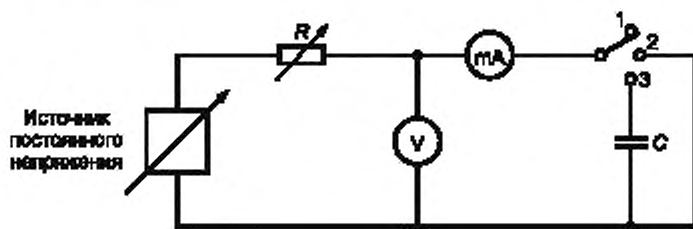
Рисунок 1 — Испытательная установка для выдержки при постоянном напряжении
