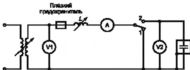
Рисунок 2 — Испытательная установка для разрушающего испытания переменным напряжением
