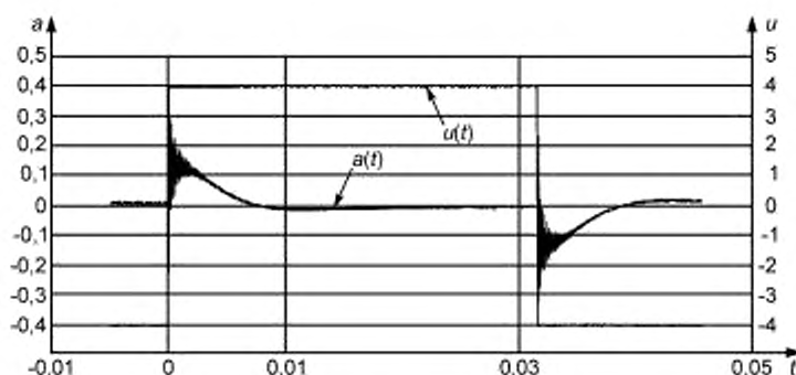
Рисунок С.3 — Входной и выходной сигналы, используемые для расчета передаточной функции вибростенда
