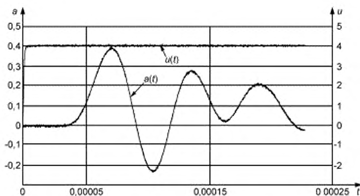
Рисунок С.6 — Отклик вибростенда в области высоких частот
