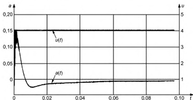
Рисунок С.4 — Отклик вибростенда в области низких частот
