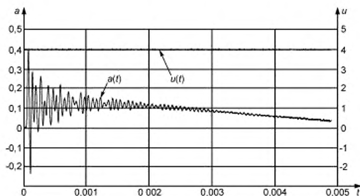
Рисунок С.5 — Отклик вибростенда в области средних частот
