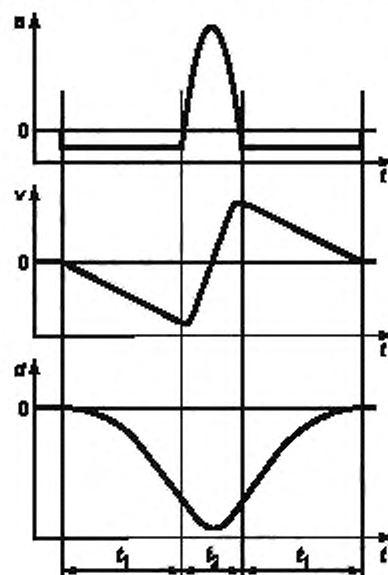
a — ускорение ударного импульса; v — скорость; d — перемещение; t — время; t_1 — длительность предударного (последударного) импульса; t_2 — длительность импульса (основной части)
