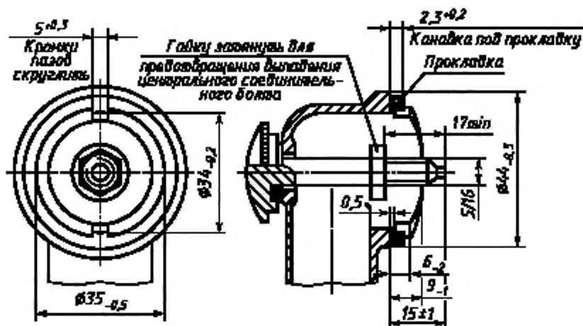
Рисунок 1 — Соединительное колено AA
