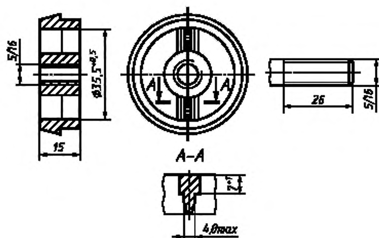
Рисунок 5 — Резьбовая втулка АВ
