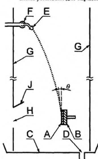
Рисунок А.1 — Схема установки для определения показателей световозвращения при дождевании
