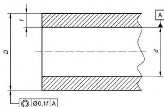
Рисунок 1 — Наружный и внутренний диаметры трубы
