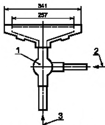
а — одиночная горелка, используемая при стандартной лестнице
