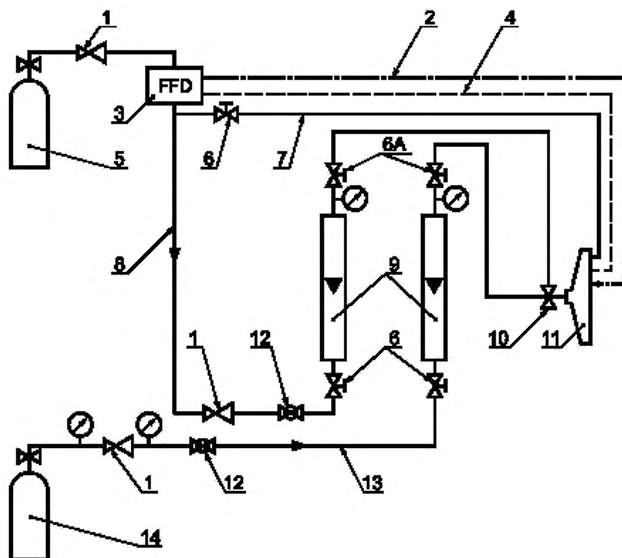
1 — регулятор; 2 — пьезоэлектрический воспламенитель; 3 — устройство для прерывания работы горелки; 4 — контрольные термодатчики; 5 — баллон с пропаном; 6 — винтовой клапан (6А — альтернативное расположение); 7 — вспомогательное питание; 8 — поступление газа; 9 — расходомер типа ротаметра; 10 — смеситель Вентури; 11 — горелка; 12 — шариковый клапан; 13 — поступление воздуха; 14 — баллон со сжатым воздухом
