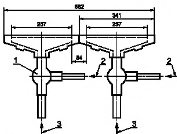
б — комбинация двух горелок, используемая при широкой лестнице
