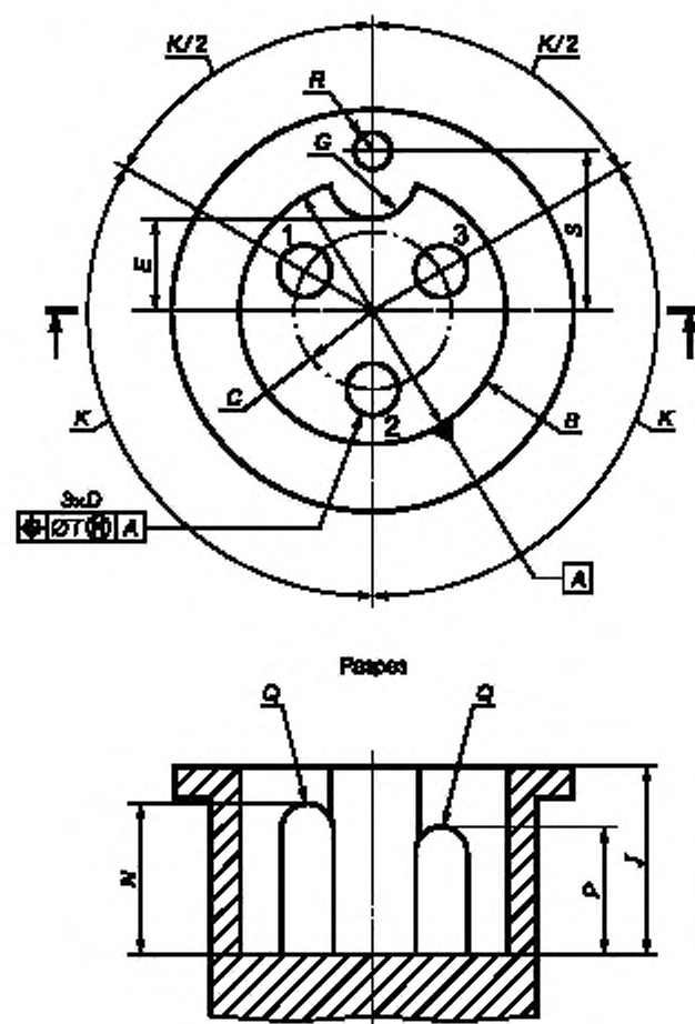
Рисунок А.7 — Трехконтактная розетка
