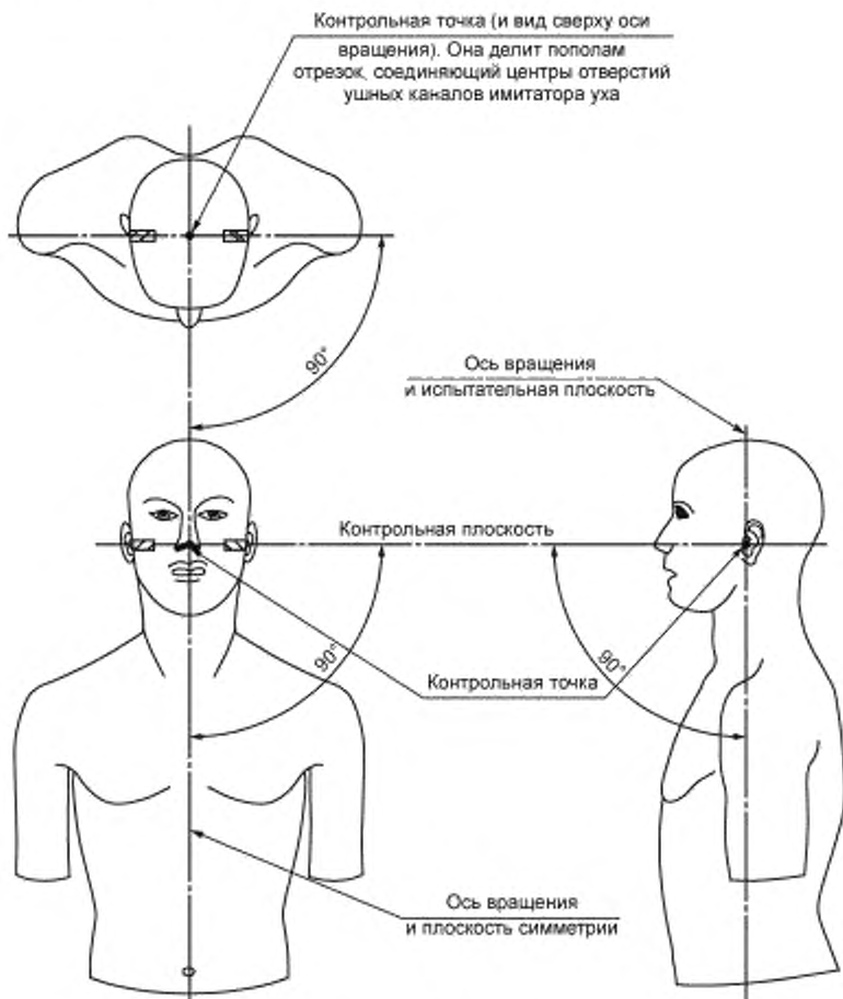
Рисунок С.1 — Геометрические характеристики манекена
