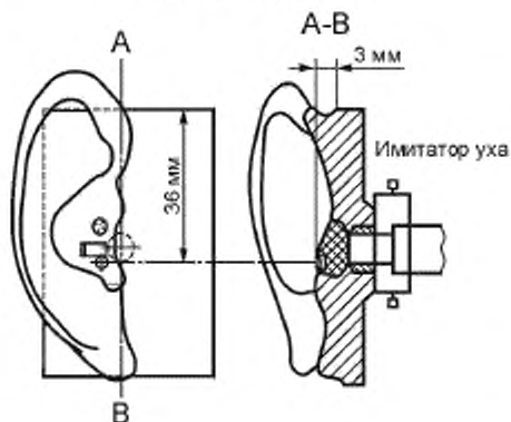
Положение микрофона при входе звука, манекен KEMAR (правое ухо)
