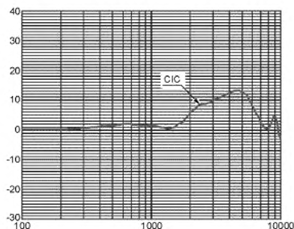
Рисунок А.4 — Положение микрофона и соответствующая переходная характеристика микрофона полностью внутриканального слухового аппарата в свободном поле
