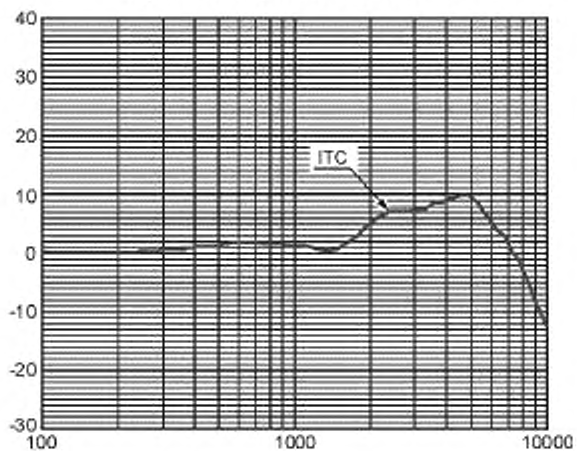
Переходная характеристика микрофона внутриканального слухового аппарата в свободном поле
