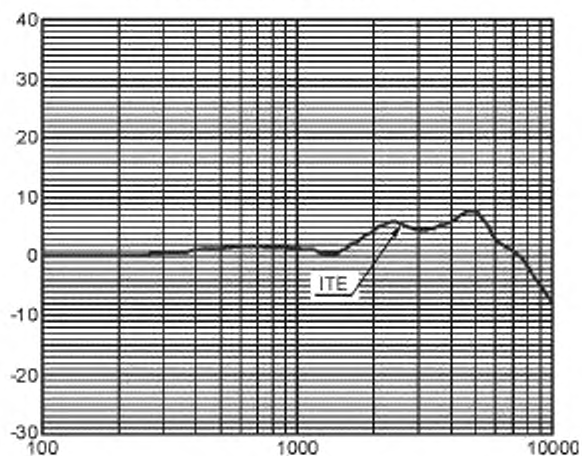
Переходная характеристика микрофона внутриушного слухового аппарата в свободном поле
