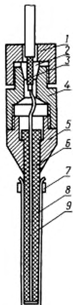
1 — зажимная гайка; 2 — сухари; 3 — кабель; 4 — нажимная гайка; 5 — корпус; 6 — изоляционный стержень; 7 — зажимное кольцо; 8 — пленочный электрет; 9 — электрод
