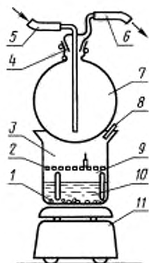
Установка для ускоренного старения в водяном паре
