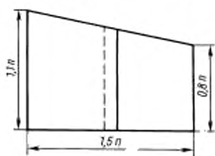
Схема реверберационной камеры
