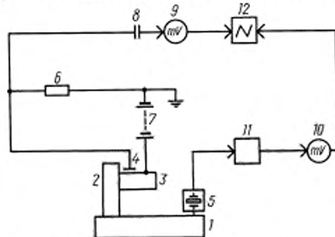
1 — стенд вибростенда; 2 — приспособление для испытаний; 3 — испытуемое изделие; 4 — искусственный электрод; 5 — пьезоэлектрический вибропреобразователь; 6 — резистор с номинальным сопротивлением 2—5 МОм; 7 — батарея элементов; 8 — конденсатор; 9, 10 — милливольтметры; 11 — катодный повторитель; 12 — осциллограф
