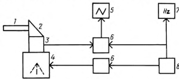
1 — испытуемое изделие; 2 — согласующий держатель; 3 — пьезоэлектрический детектор резонансных частот; 4 — вибратор; 5 — индикатор (осциллограф); 6 — усилитель; 7 — частотомер; 8 — генератор звуковых частот
