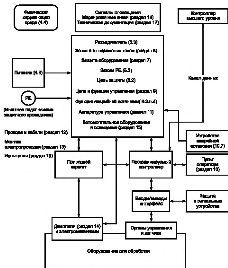
Рисунок 1 — Функциональная схема типовой машины
