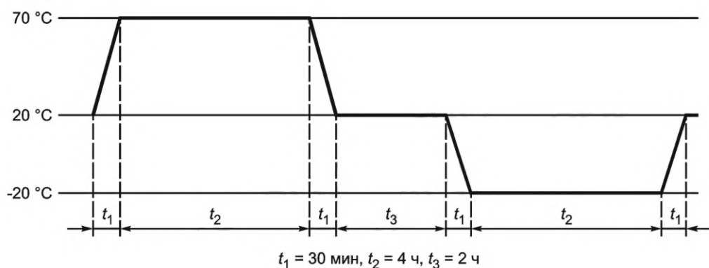
Рисунок 2 — Процедура термоциклирования
