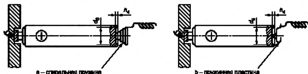
Рисунок В.12 — Примеры отрицательных контактов
