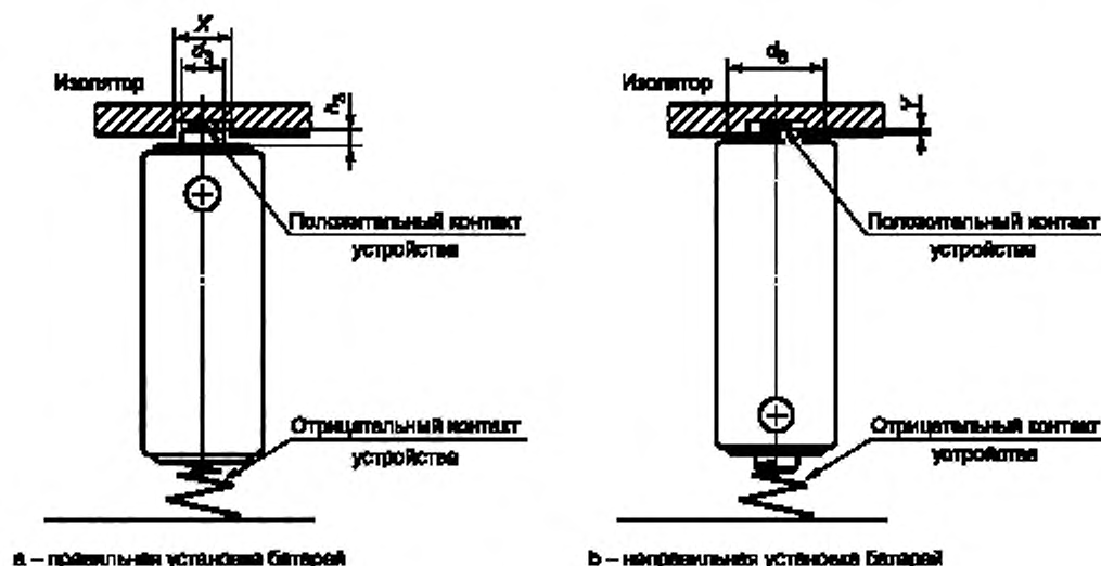
Рисунок В.6 — Пример конструкции положительного контакта оборудования
