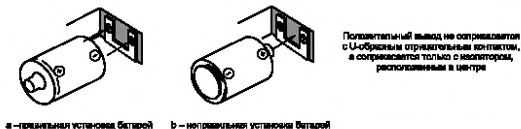
Рисунок В.4 — Отрицательный контакт U-образной формы, обеспечивающий невозможность контакта с положительным выводом батареи
