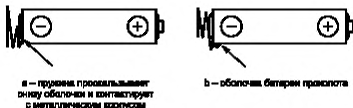
Рисунок В.10 — Примеры перекашивания пружин
