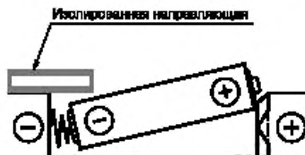
Рисунок В.11 — Один из примеров защищенной установки
