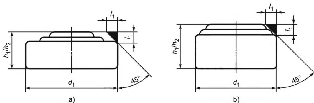
Рисунок 2 — Форма батареи
