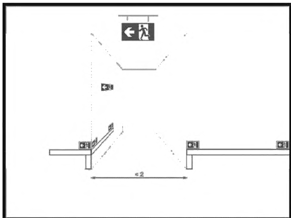
Рисунок А.4 — Примерный план разметки туликового коридора шириной не более 2 м
