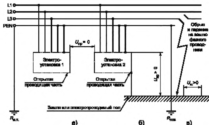
Рисунок Г.4 — Сеть TN-C с замыканием на землю, например с оборванным и упавшим на землю фазным проводом
