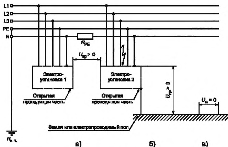
Рисунок Г.6 — Сеть TN-S с однофазным замыканием на корпус
