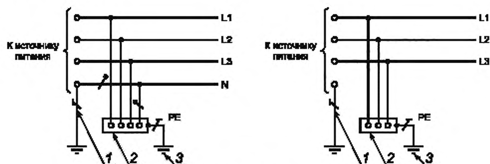
а) переменного тока
