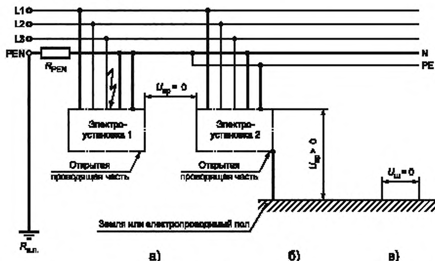
Рисунок Г.9 — Сеть TN-C-S с однофазным замыканием на корпус до точки разделения PEN-проводника на N- и PE-проводники
