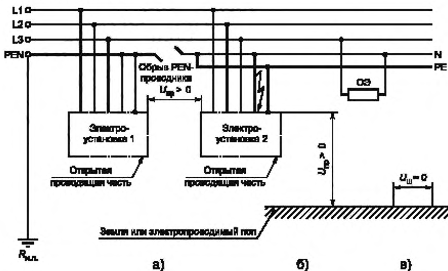
Рисунок Г.7 — Сеть TN-C-S с обрывом PEN-проводника
