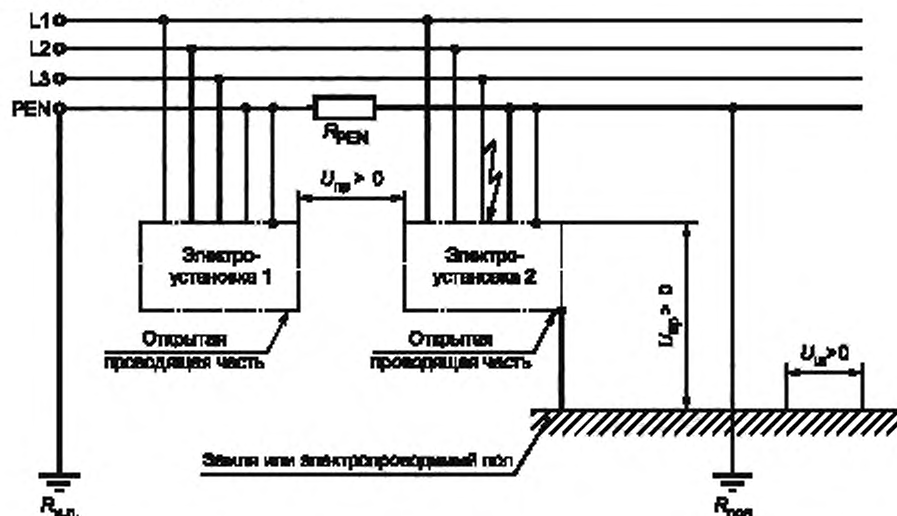
Рисунок Г.3 — Сеть TN-C с однофазным замыканием на корпус
