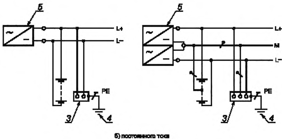
Рисунок Б.4 — Система IT переменного и постоянного тока
