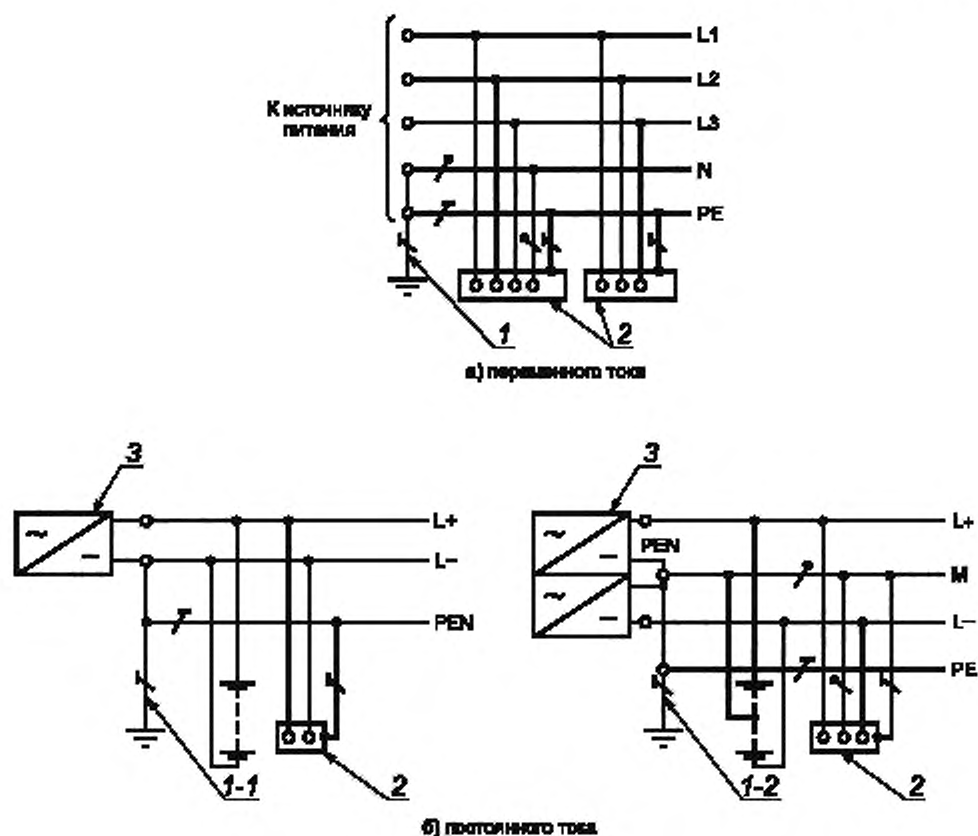
Рисунок Б.2 — Система TN-S переменного и постоянного тока
