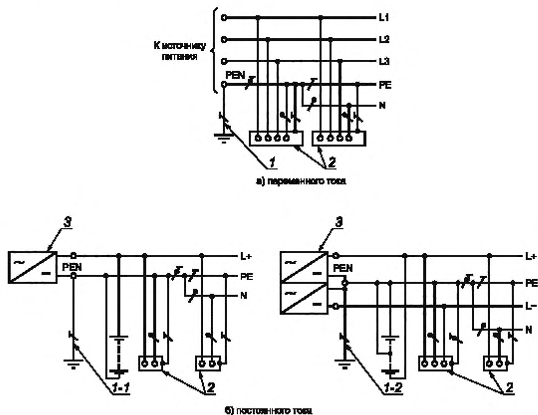
Рисунок Б.3 — Система TN-C-S переменного и постоянного тока
