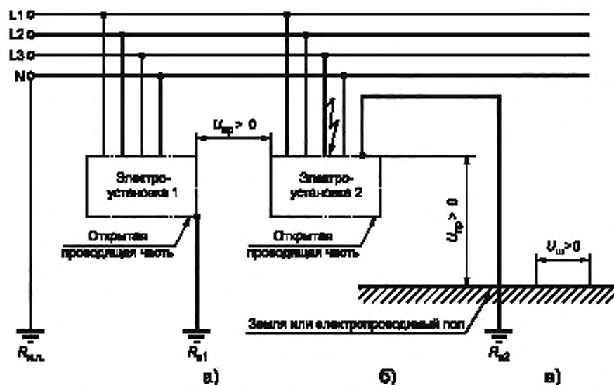
Рисунок Г.10 — Сеть ТТ с нулевым рабочим проводником с однофазным замыканием на корпус
