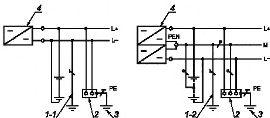
б) постоянного тока
