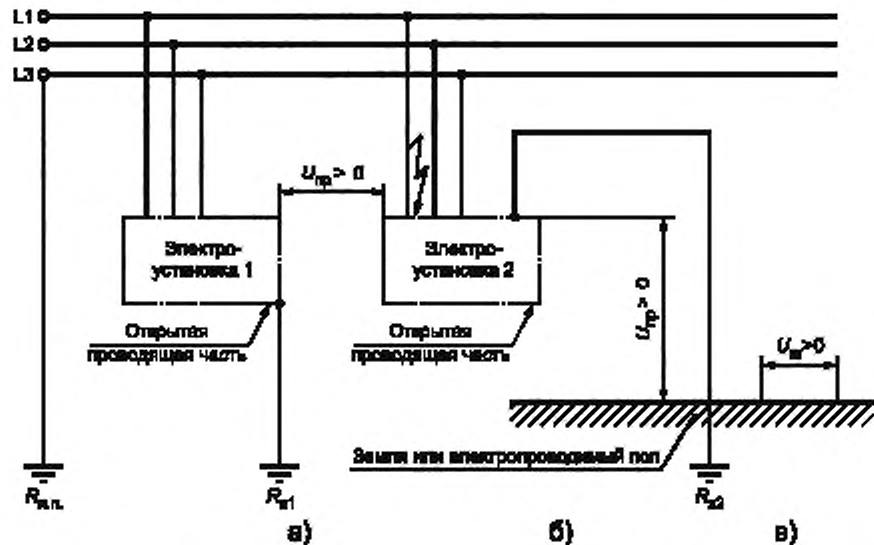
Рисунок Г.11 — Сеть ТТ без нулевого рабочего проводника с однофазным замыканием на корпус
