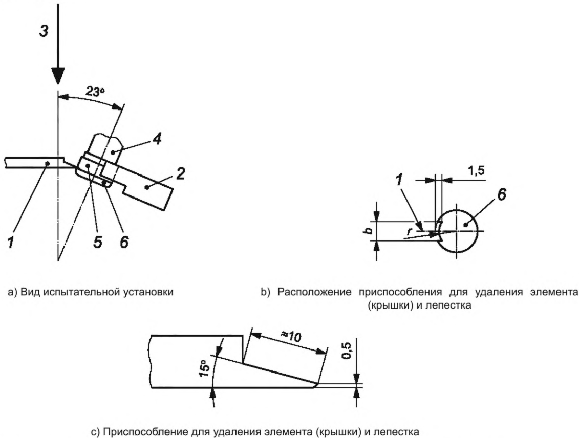
1 — приспособление для удаления (крышки) и лепестка; 2 — зажимы тисков; 3 — направление усилия отрыва; 4 — флакон; 5 — алюминиевый колпачок; 6 — пластмассовый элемент (пластмассовая крышка)
