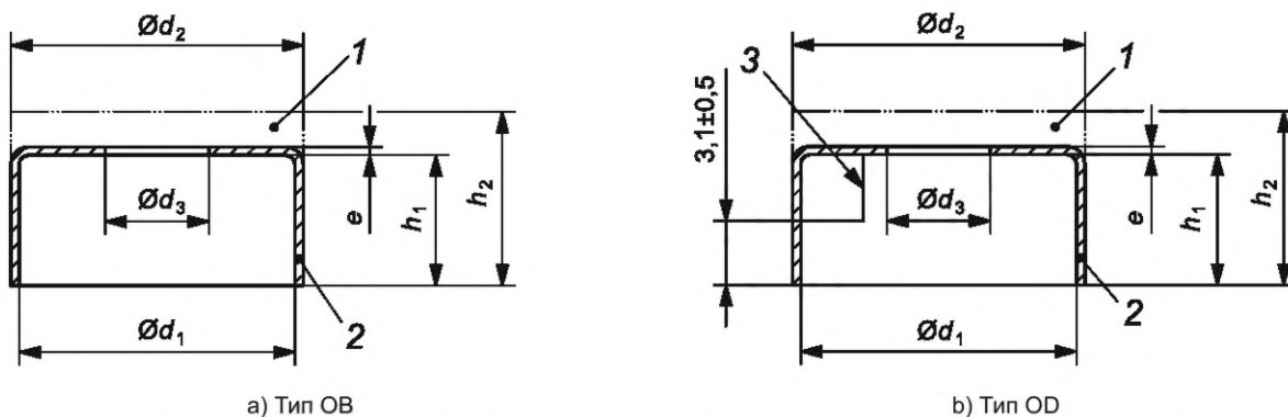
1 — пластмассовый элемент (пластмассовая крышка); 2 — алюминиевый колпачок по ИСО 8362-3; 3 — линия отметки (отрыва)
