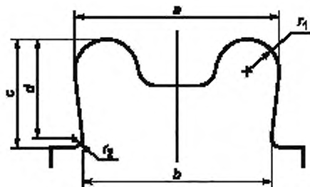
Рисунок 2 — Кнопка
