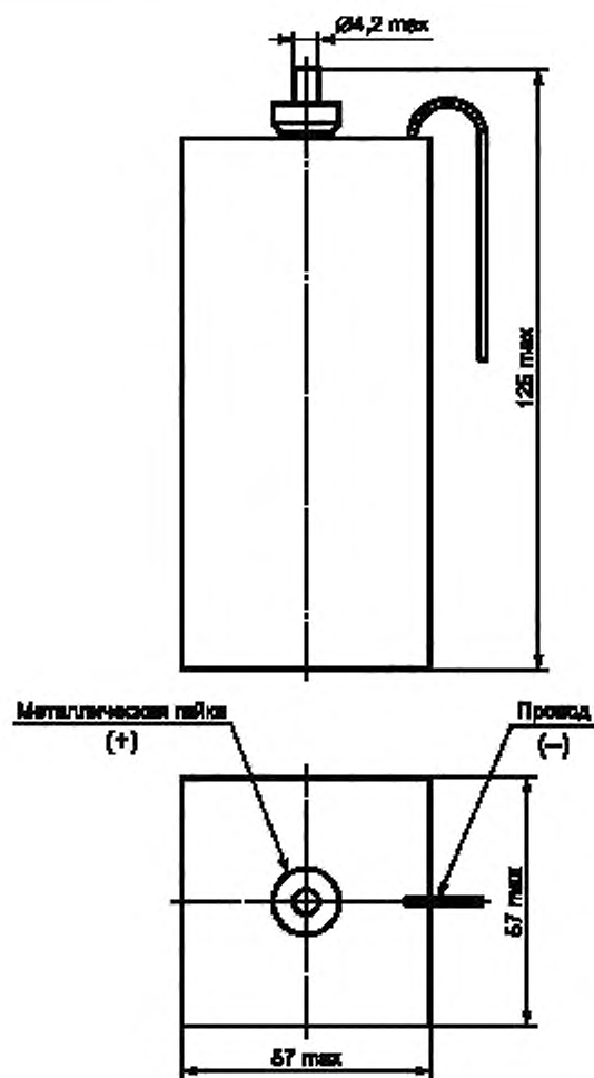
Рисунок 9 — Размеры батареи S4
