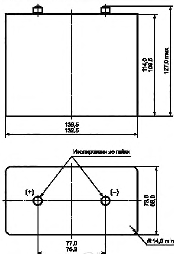
Рисунок 17 — Размеры батарей 4R25-2, 4LR25-2
