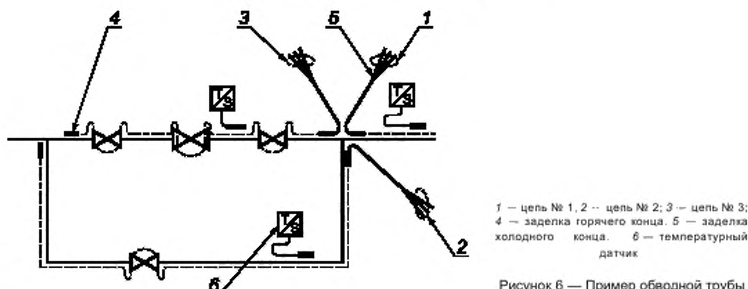
Рисунок 6 — Пример обводной трубы
