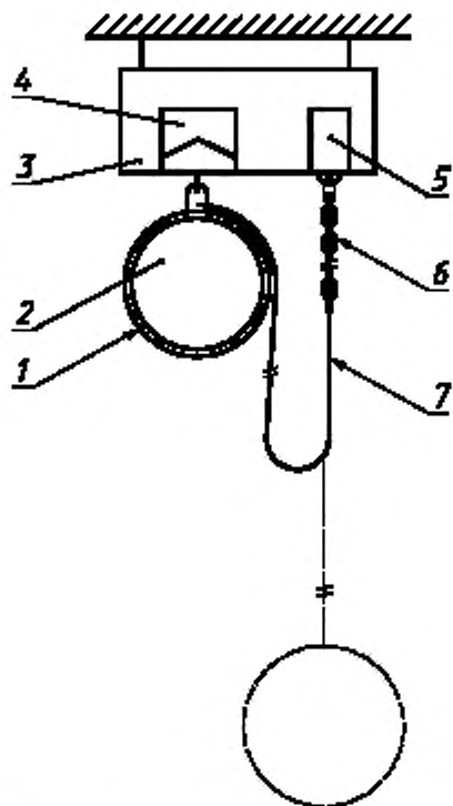
1 — пояс; 2 — груз или манекен массой 100 кг; 3 — подъемное устройство; 4 — расцепляющее устройство; 5 — датчик измерительного устройства; 6 — технологический фал для удлинения стропы до 2 м или до двух длин стропы; 7 — стропа
