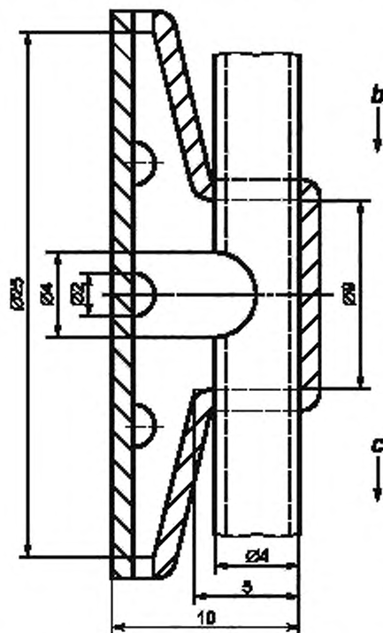
а — прозрачный материал; б — осушающий воздух, в — проба с осушающим воздухом
