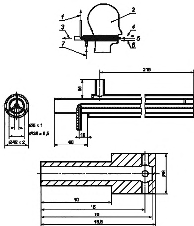
1 — трубка для подключения манометра, 2 — голова манекена; 3 — «дыхательной машины» вдыхаемый воздух; 4 — выдыхаемый воздух; 5 — трубка для измерения давления, 6 — вдыхаемый воздух; 7 — от дыхательной машины, выдыхаемый воздух
