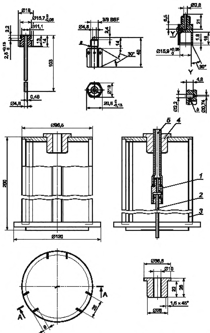
Рисунок 3 — Типовая схема устройства распылителя
