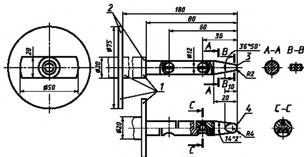
1 — изоляционный материал; 2 — столонная плата; 3 — цилиндр; 4 — сфера
