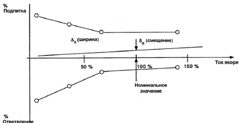
Рисунок 5 – Зона безыскровой коммутации при постоянной скорости вращения
