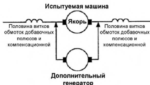
Рисунок 4 – Дополнительный генератор, используемый для увеличения или отведения части тока якоря
