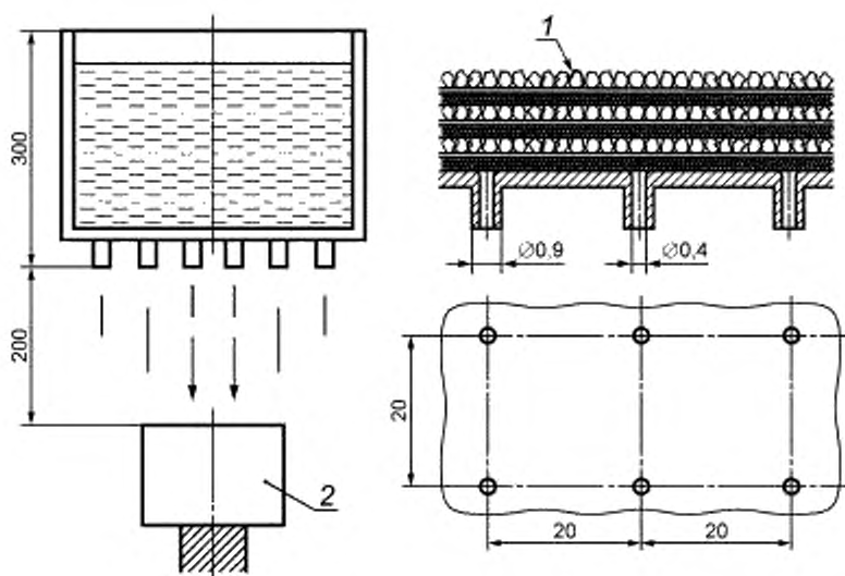
1 — слой песка и гравия для регулирования потока воды, эти слой разделены металлической сеткой и промокающей бумагой; 2 — испытуемая машина
