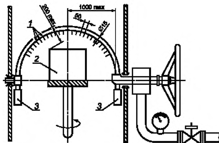
1 — отверстия диаметром 0,4 мм (показаны отверстия для капель воды для проверки степени защиты второй характеристической цифры 2); 2 — испытуемая машина; 3 — противовес
