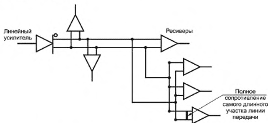
Рисунок 9 — Организация линии передачи в форме гирляндной цепи
