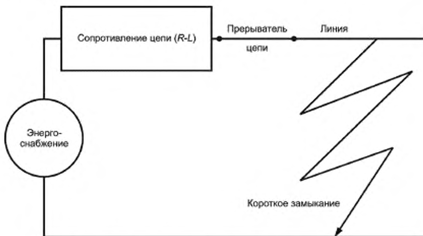
Рисунок А.1 — Эквивалентная электрическая цепь сети
