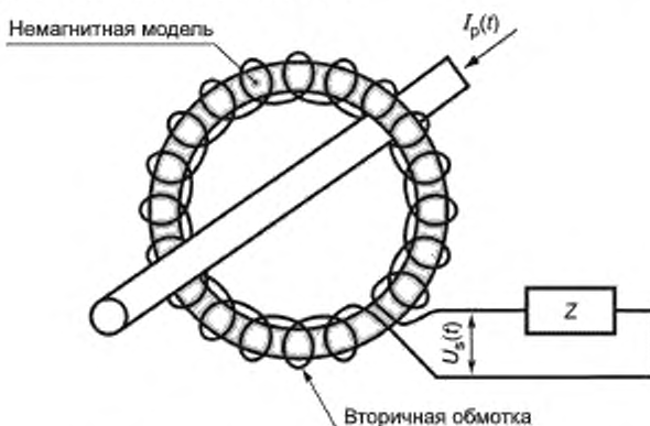
Рисунок С.4 — Автономная катушка без сердечника
