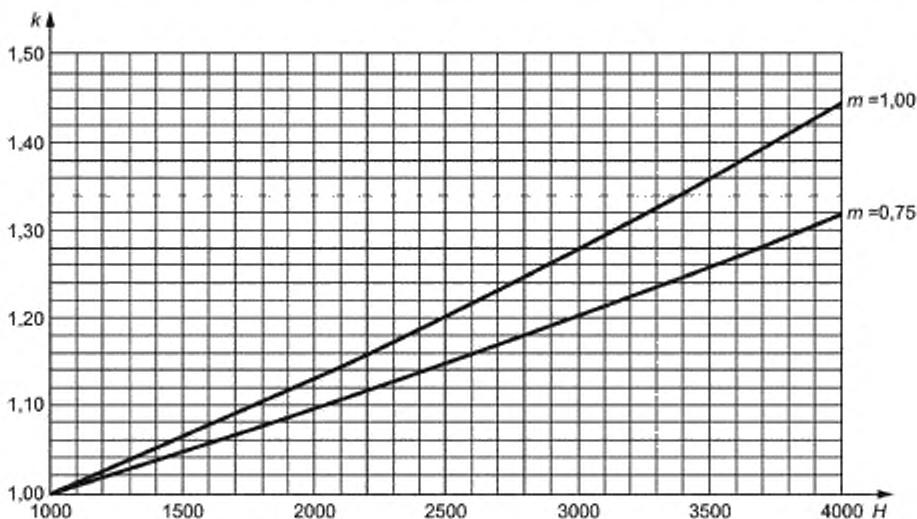
Рисунок 3 — Корректирующий высотный коэффициент
