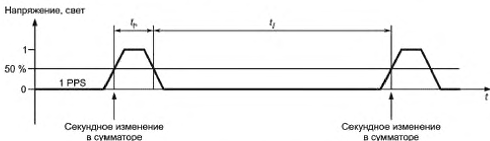
Рисунок 14 — Форма синхроимпульса
