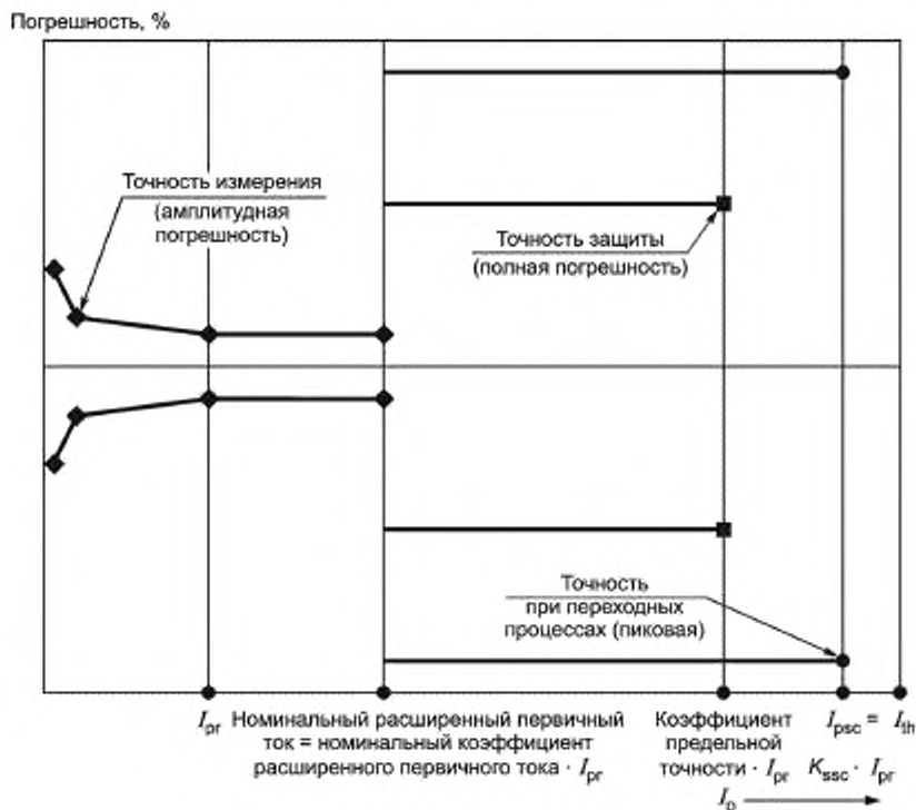
Рисунок Е.1 — Пределы точности многоцелевого ЭТТ
