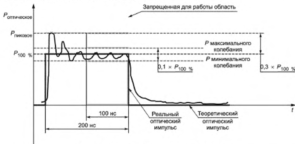
Рисунок 5 — Характеристики оптического импульса
