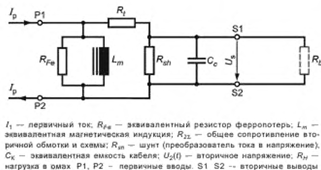
Рисунок С.3 — Эквивалентная цепь трансформатора тока с ферродинамическим сердечником с напряжением на выходе
