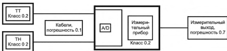
Традиционная измерительная система
