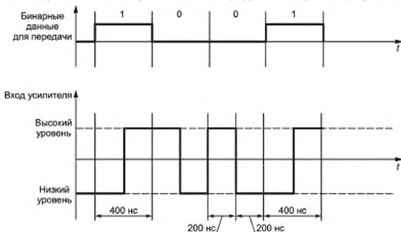
Рисунок 4 — Манчестерское кодирование
