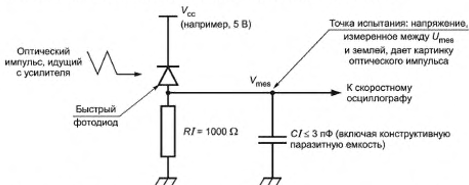
Рисунок 6 — Испытательная цепь для определения параметров оптического импульса
