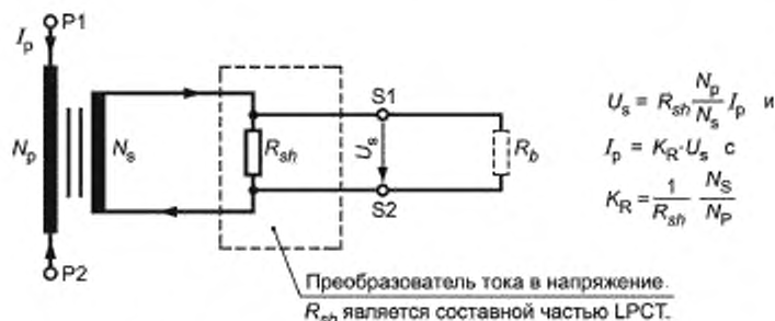
Рисунок С.2 — Трансформатор с ферродинамическим сердечником
