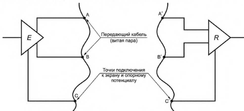
Рисунок 7 — Интерфейс с медно-проволочными линиями
