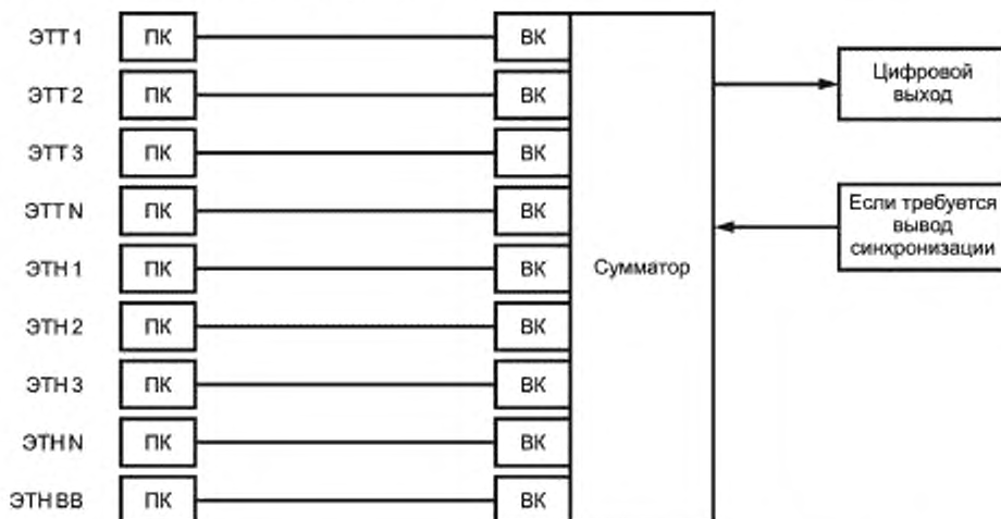
Рисунок В.1 — Объединение ЭТТ и ЭТН для создания цифрового выхода
