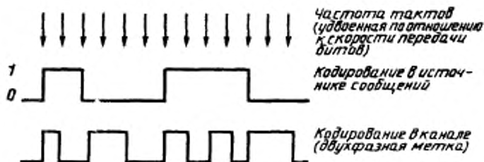
Кодирование канала
