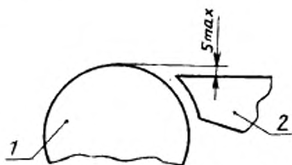
1 — пильный диск; 2 — расклинивающий нож
