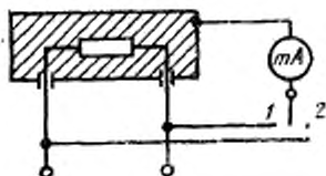
Рисунок 4 — Схема измерения тока утечки при рабочей температуре для остальных однофазных машин (кроме класса II)
