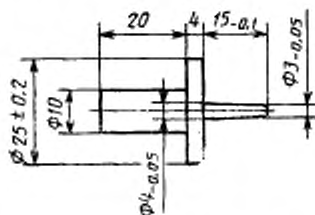
Рисунок 2 — Испытательный шуп
