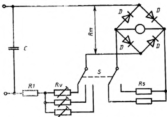
Рисунок 1A1 — Схема цепи для измерения тока утечки
