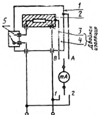
Рисунок 2 — Испытательный шуп
