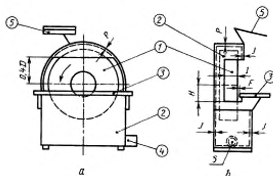
1 — шлифовальный круг; 2 — защитный кожух круга; 3 — рабочий упор; 4 — мундштук для удаления пыли; 5 — прозрачный экран; P — толщина периферической части кожуха; F — толщина боковых стенок кожуха; 5 — внутреннее сечение мундштука; D — максимальный наружный диаметр круга; J — зазор между рабочим упором и кругом; L — толщина круга
