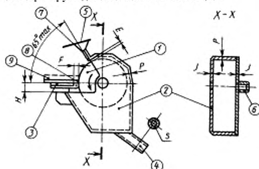
1 — шлифовальный круг, 2 — защитный кожух круга, 3 — рабочий упор, 4 — щетка для удаления пыли, 5 — прозрачный экран, 6 — ось регулировки, 7 — искрогаситель, 8 — рабочая зона круга, 9 — обрабатываемое изделие; H — толщина периферической части кожуха, J — толщина боковых стенок кожуха, S — внутреннее сечение монтажного; D — максимальный наружный диаметр круга, E — зазор между искрогасителем и кругом, F — зазор между рабочим упором и кругом
