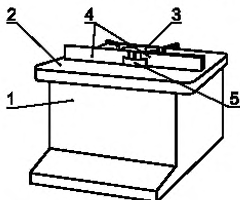
1 — опора; 2 — стол; 3 — режущий узел; 4 — направляющая; 5 — отражение режущего инструмента
