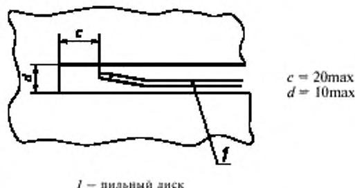
Рисунок 104 — Размеры прорези в столе
