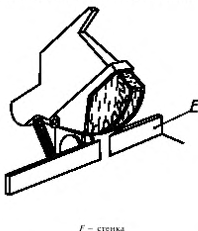
Рисунок 102 — Защитный кожух открытой конструкции
