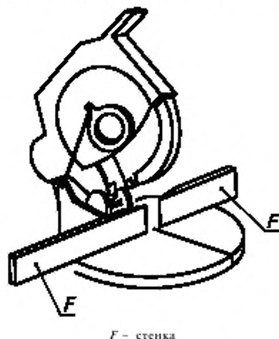
Рисунок 101 — Защитный кожух U-образной конструкции
