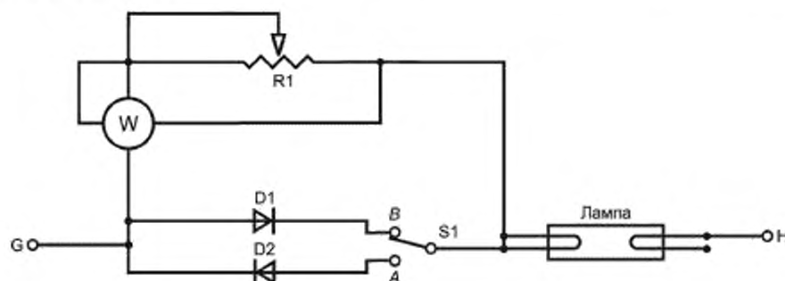
Рисунок Н.2 — Схема испытания асимметричной мощностью
