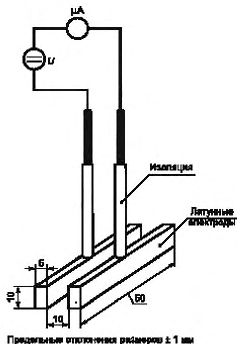
Рисунок 1 — Испытательная установка для определения диэлектрических свойств заполнителя
