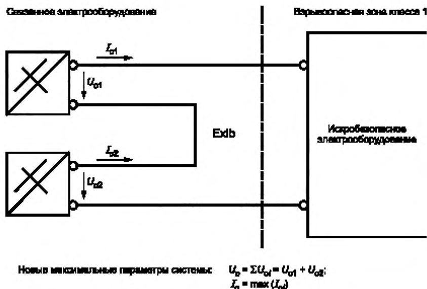
Рисунок В.1 — Последовательное соединение. Суммирование значений напряжения
