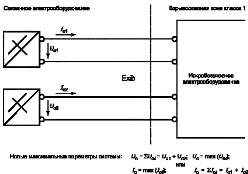
Рисунок В.3 — Последовательные и параллельные соединения. Суммирование значений напряжения и тока
