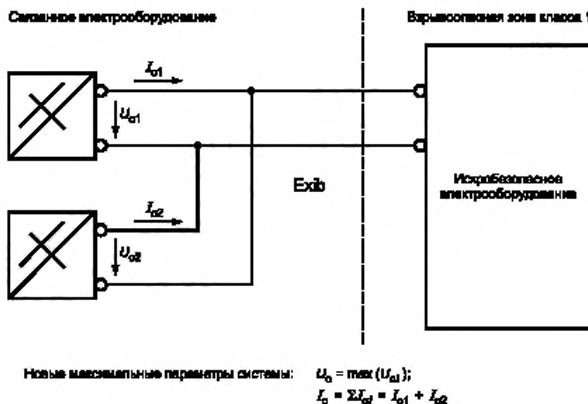
Рисунок В.2 — Параллельное соединение. Суммирование значений тока
