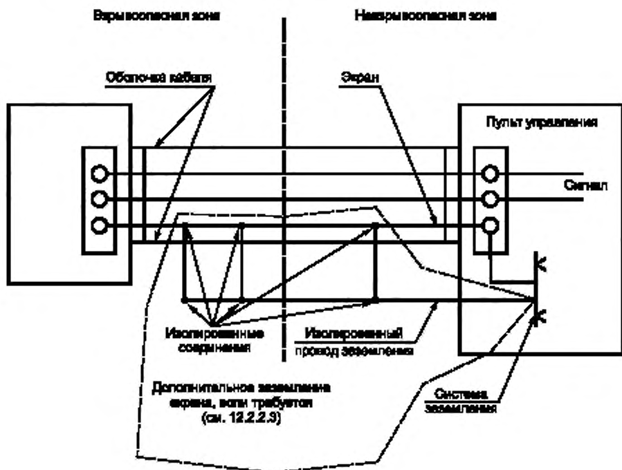
Рисунок 3 — Заземление проводящих экранов
