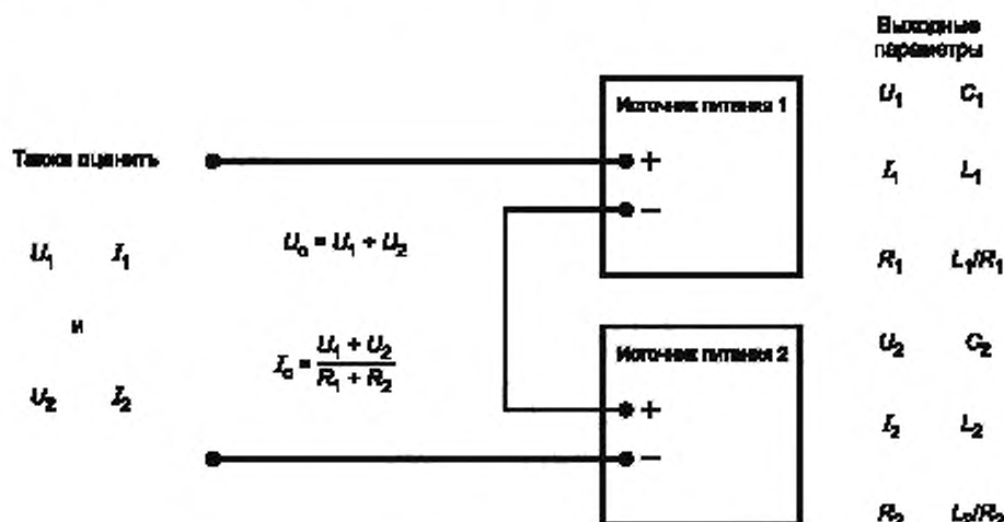
Рисунок В.1 — Источники питания, подключенные последовательно
