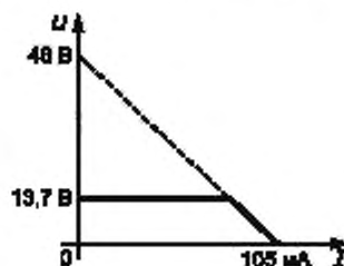
Рисунок С.3а — Выходные характеристики
