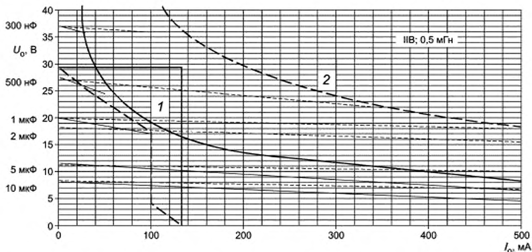
Рисунок С.6а — Сложение значений тока
