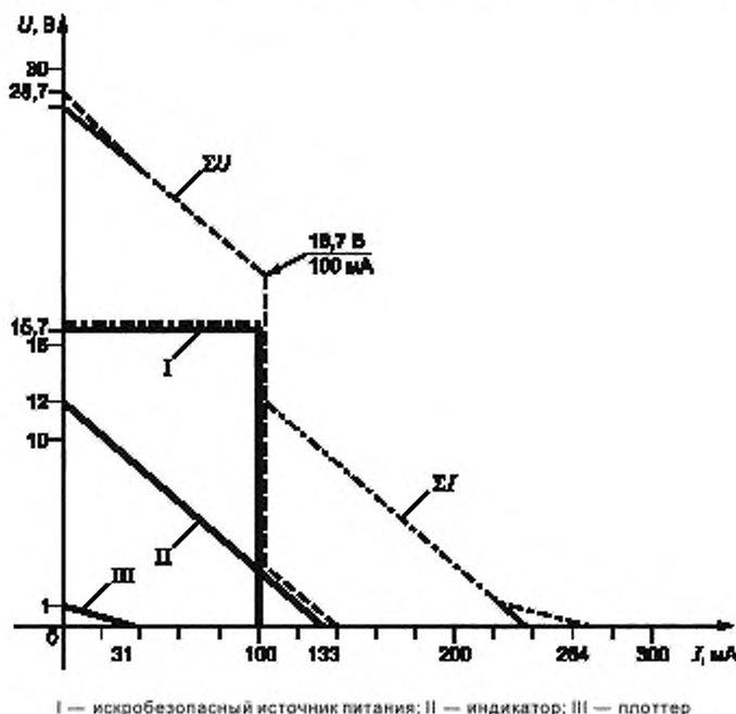
Рисунок С.5 — Суммарные характеристики цепи, представленной на рисунке С.4
