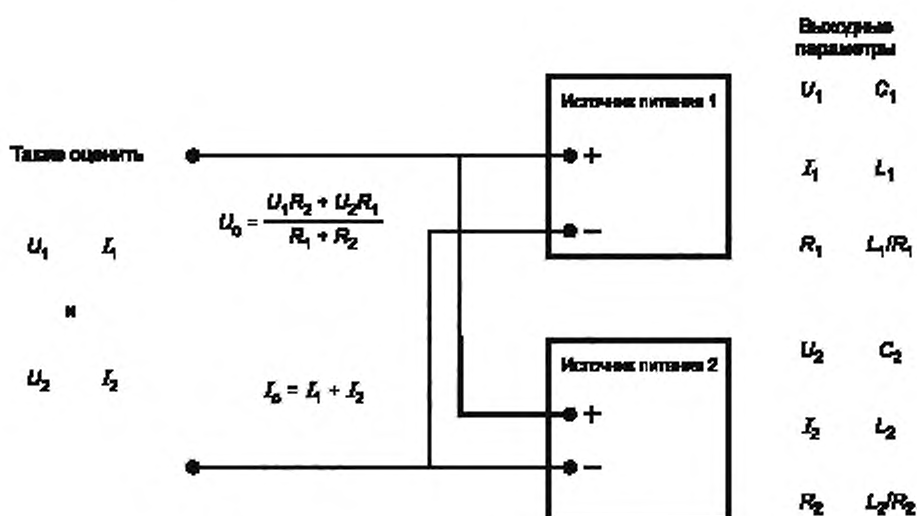
Рисунок В.2 — Источники питания, подключенные параллельно
