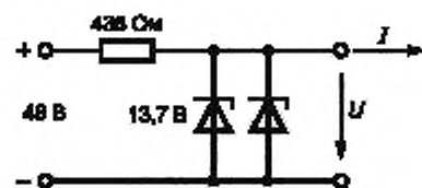
Рисунок С.3b — Эквивалентная цепь
