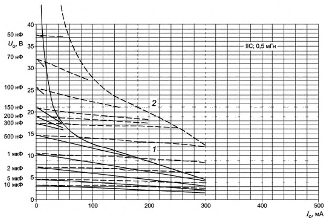
Рисунок С.7b — Диаграмма для значения 0,5 мГн (продолжение)
