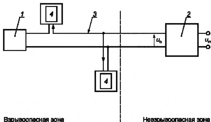
1 — сертифицированное искробезопасное оборудование; 2 — сертифицированное связанное искробезопасное оборудование; 3 — кабель; 4 — простое электрооборудование
