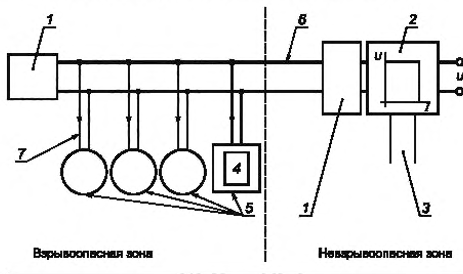
1 — оконечное устройство; 2 — источник питания; 3 — данные; 4 — ручной терминал; 5 — полевые устройства; 6 — магистральный кабель; 7 — ответительный кабель
