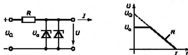
Рисунок С.1б — Трапециевидная характеристика
