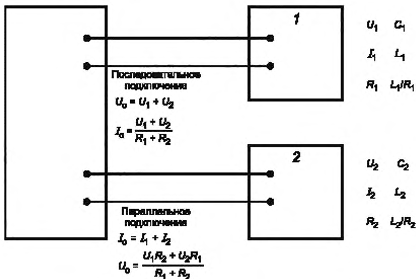
Рисунок В.3 — Произвольно подключенные источники питания
