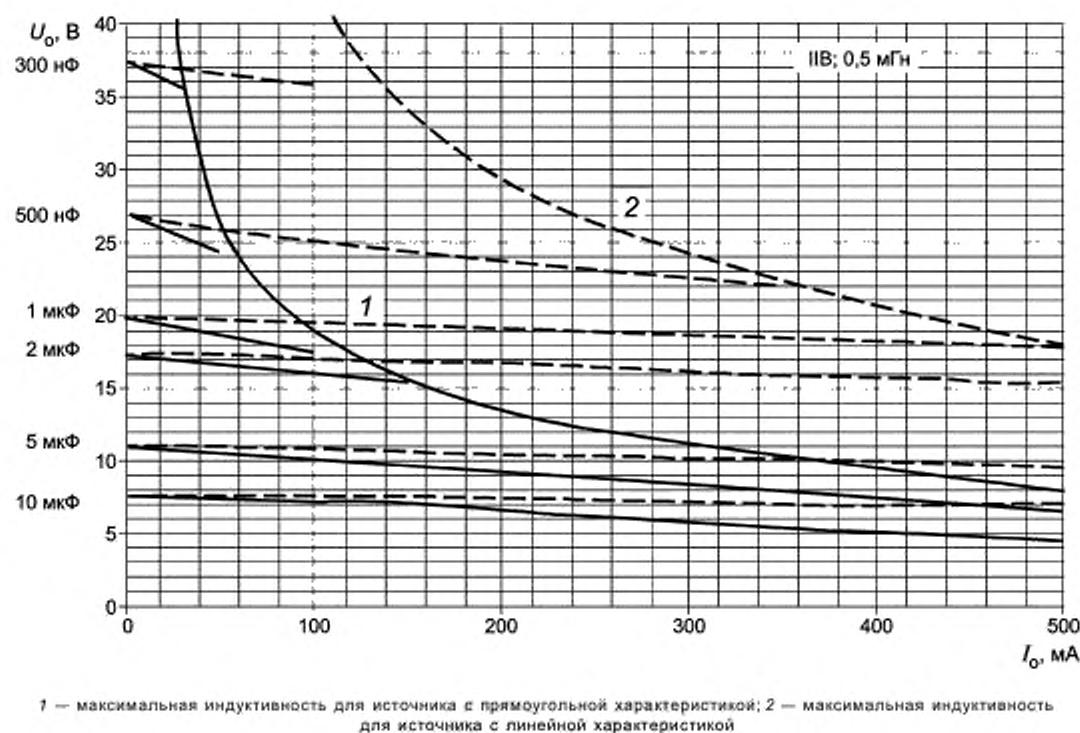
Рисунок С.8b — Диаграмма для значения 0,5 мГц (продолжение)
