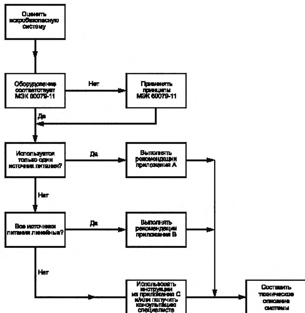
Рисунок 1 — Схема оценки системы
