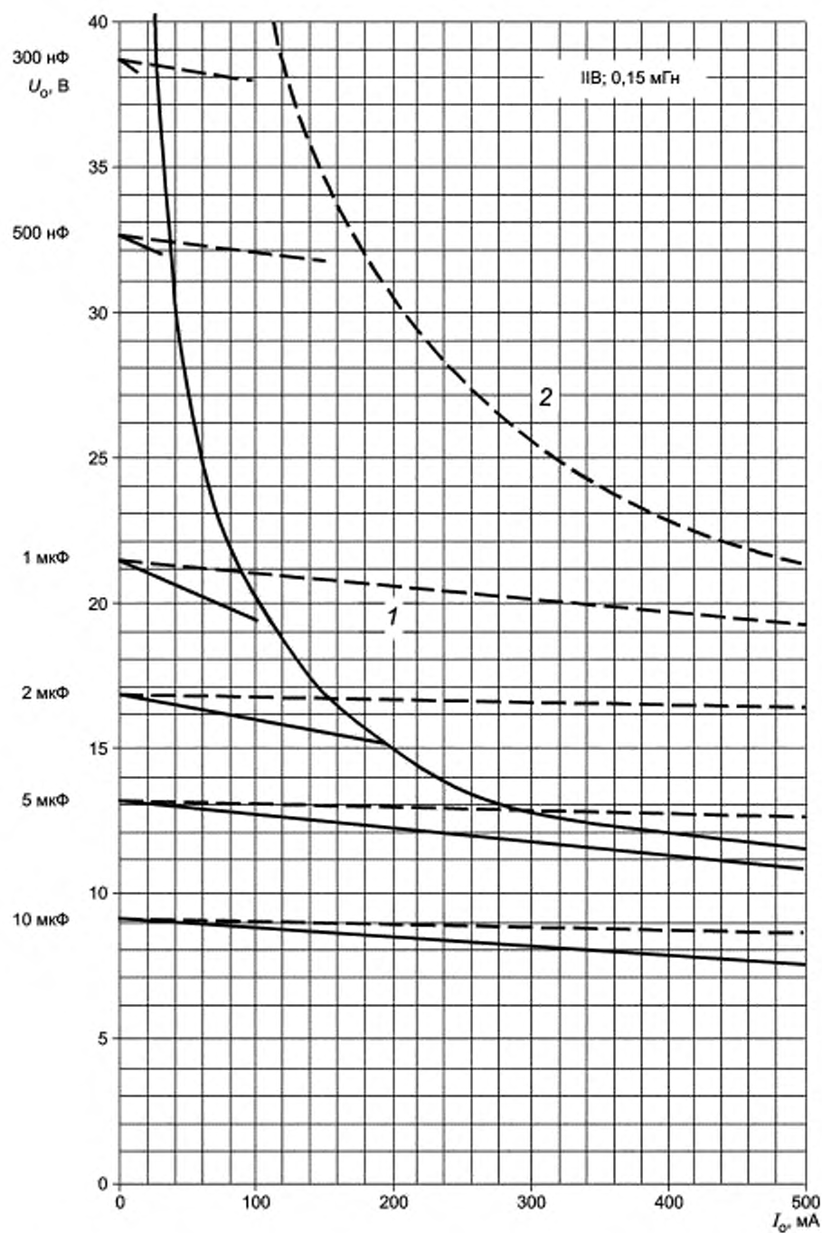
Рисунок С.8а — Диаграмма для значения 0,15 мГн
