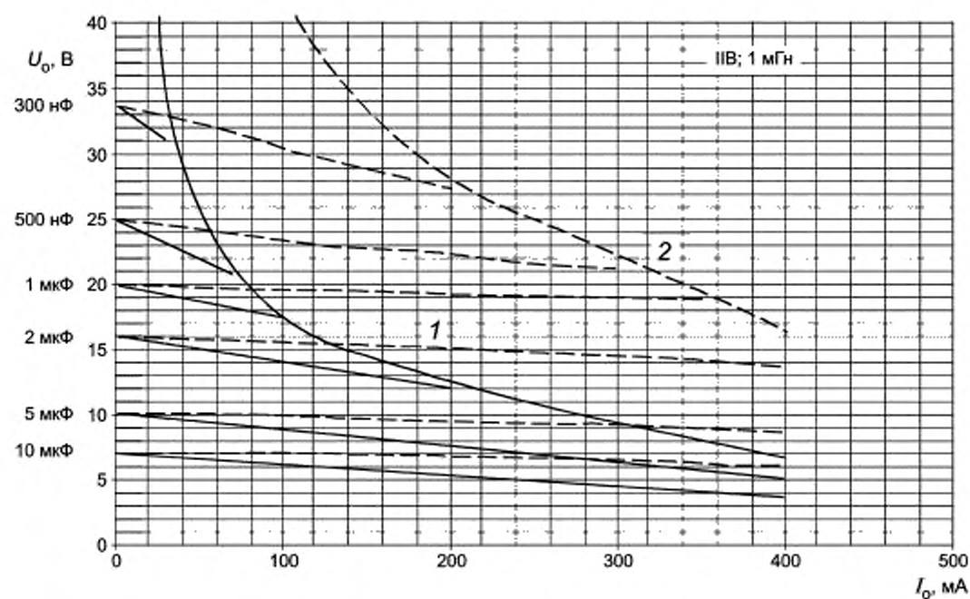
Рисунок С.8с — Диаграмма для значения 1 мГн (продолжение)
