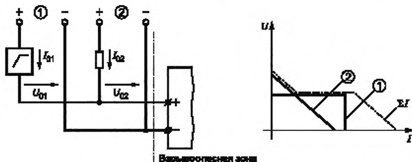
Рисунок С.2с — Параллельное подключение со сложением значений тока
