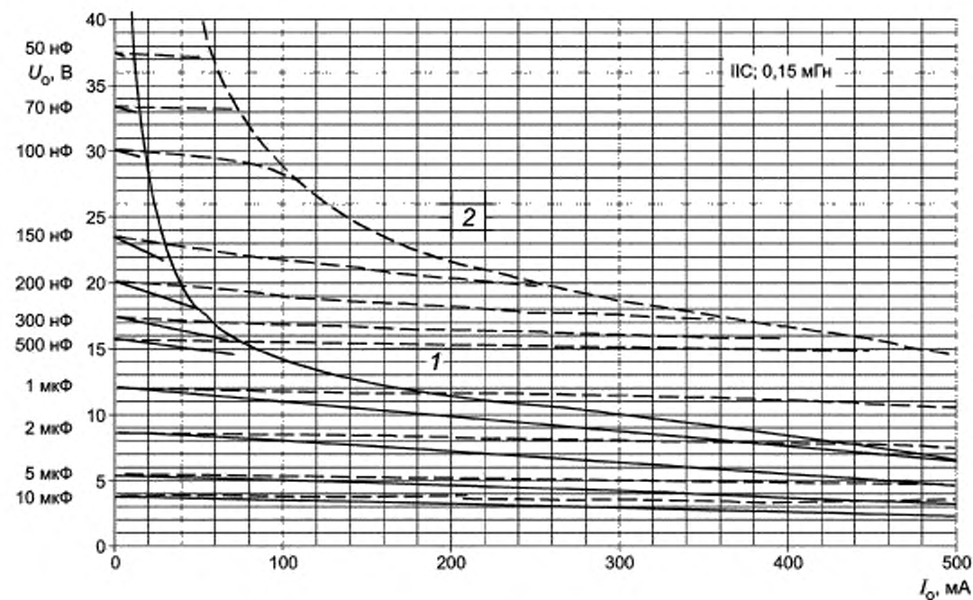
Рисунок С.7а — Диаграмма для значения 0,15 мГн (продолжение)
