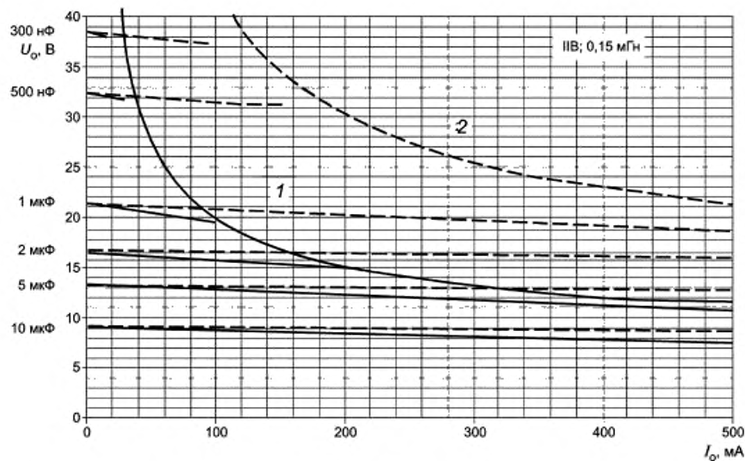
Рисунок С.8а — Диаграмма для значения 0,15 мГн (продолжение)
