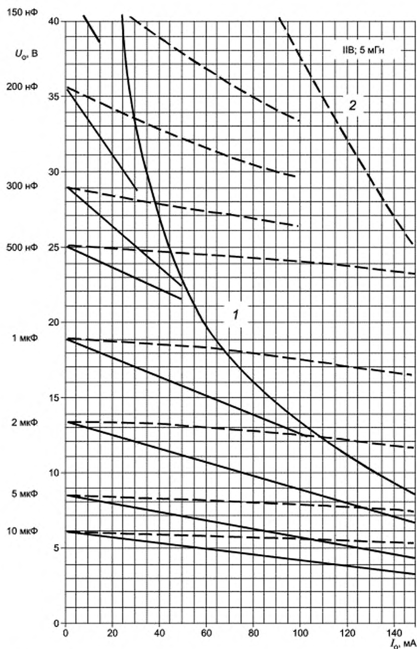
Рисунок С.8е — Диаграмма для значения 5 мГн
