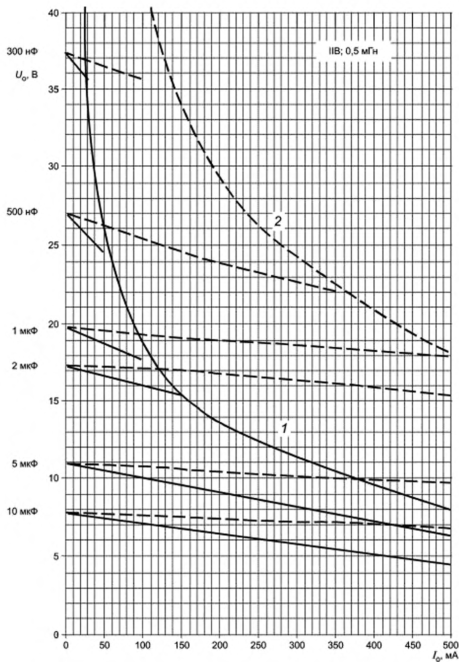
Рисунок С.8b — Диаграмма для значения 0,5 мГн
