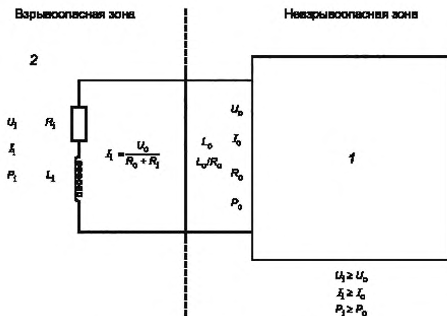
Рисунок D.1 — Типичная индуктивная цепь
