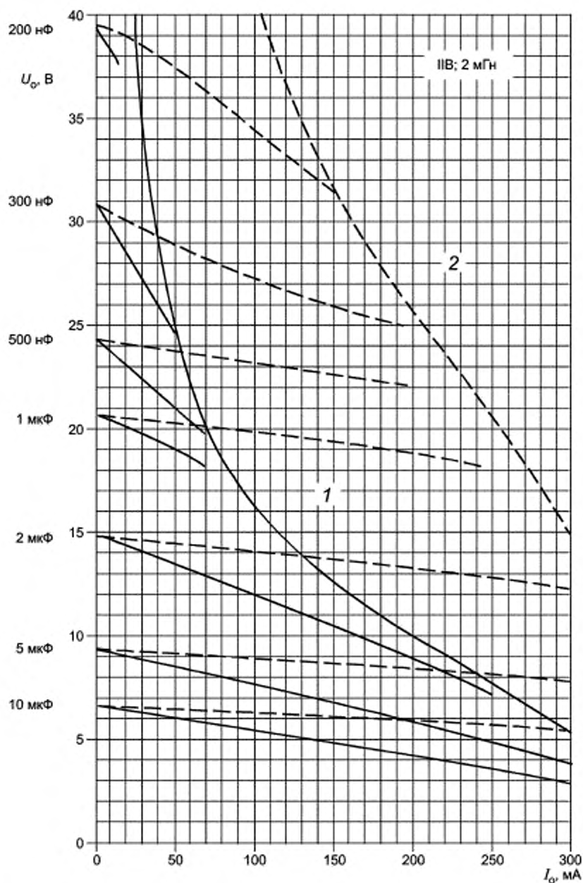
Рисунок С.8d — Диаграмма для значения 2 мГн
