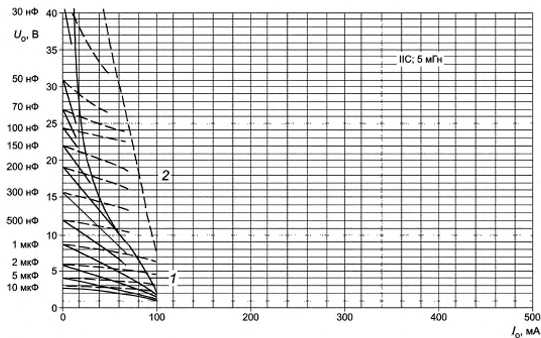
Рисунок С.7е — Диаграмма для значения 5 мГн (продолжение)
