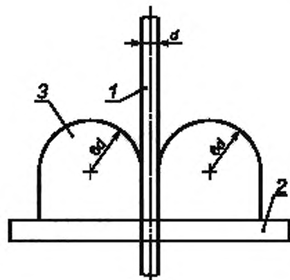
1 — образец резистивного распределенного электронагревателя, 2 — стальное основание, 3 — металлическая оправка, d — диаметр распределенного электронагревателя или первичная плоскость изгиба, если изготовитель не указал иное
