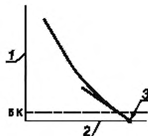
1 — температура образца минус температура воздуха в печи ( T_s - T_o ), К; 2 — температура в печи T_o , °С; 3 — зарегистрированное значение температуры T_s , °С
