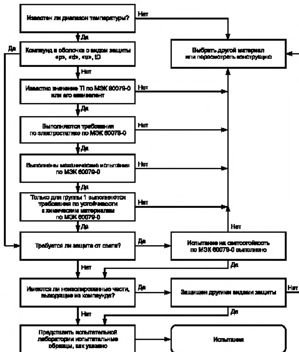
Рисунок А.1 — Основные требования к компаундам для оборудования с взрывозащитой вида «герметизация компаундом "m"»
