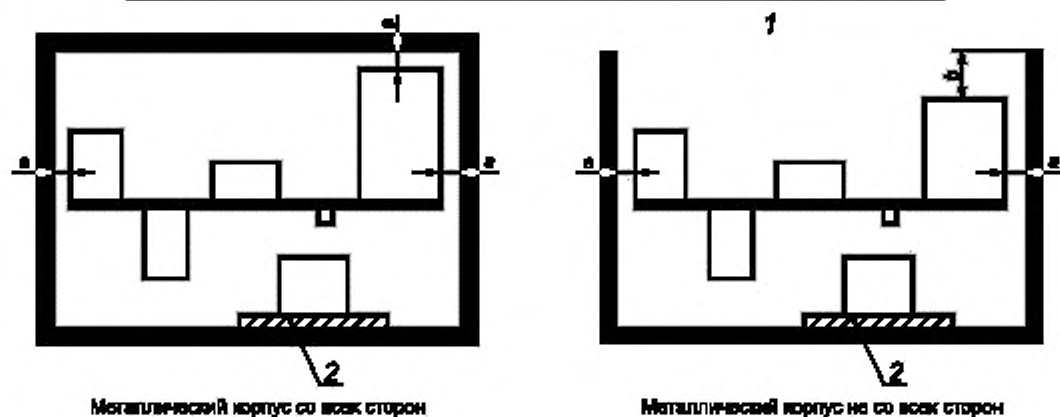
Металлический корпус со всех сторон
