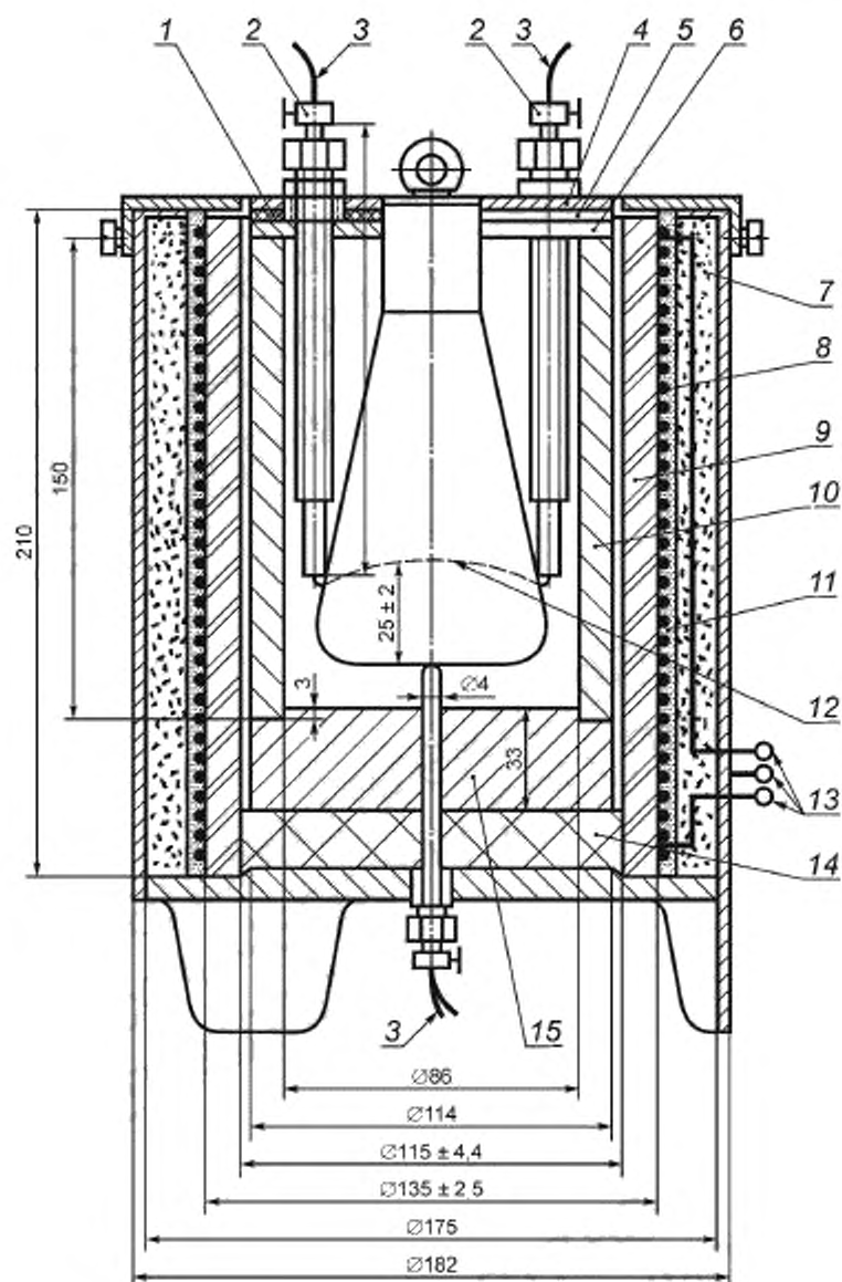
1 — высокотемпературная изоляция; 2 — зажимные втулки; 3 — термопары; 4 — верхняя часть крышки; 5 — изоляционное кольцо; 6 — нижняя часть крышки; 7 — теплоизоляция; 8 — нагреватель; 9 — керамическая трубка; 10 — стальной цилиндр; 11 — высокотемпературная мастика; 12 — контрольные точки; 13 — соединение нагревателя на напряжение 220 В; 14 — изоляционный диск; 15 — металлическое основание
