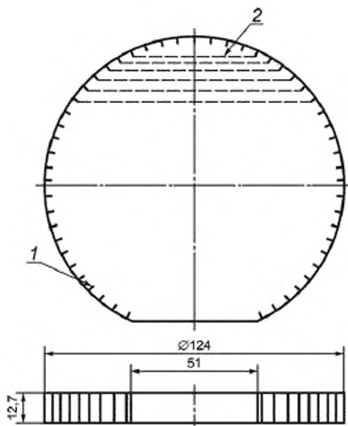
1 — паз размером 1,5×1,5 мм на боковой поверхности диска; 2 — способ укладки никель-хромового провода диаметром 0,4 мм и длиной 2,5 м
