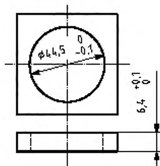
Рисунок 20 — Испытательный шаблон С
