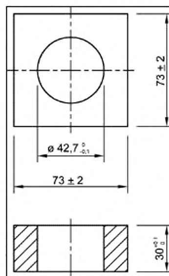
Рисунок 18 — Испытательный шаблон А
