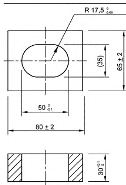
Рисунок 18 — Испытательный шаблон А
