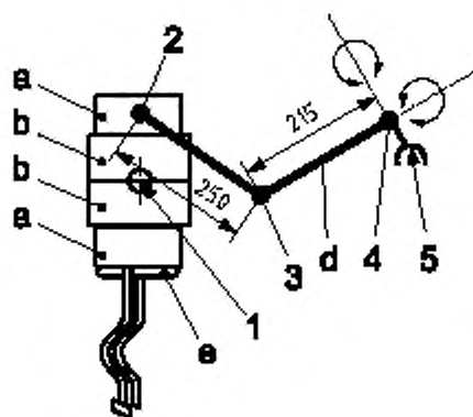
а) испытательный груз для самокатов, предназначенных для детей массой от 20 кг до 50 кг
