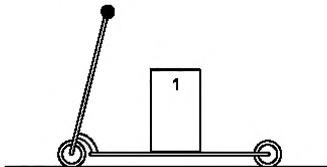
1 — испытательный груз
