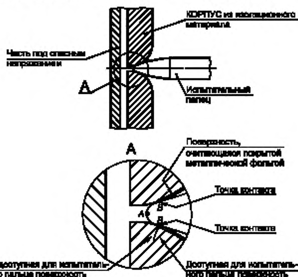
Рисунок 2 — Пример оценки УСИЛЕННОЙ ИЗОЛЯЦИИ
