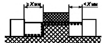
Рисунок E.6 — Неплотный стык с широкими канавками
