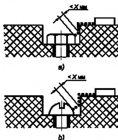
Рисунок E.8 — Промежуточная, несоединенная проводящая часть
