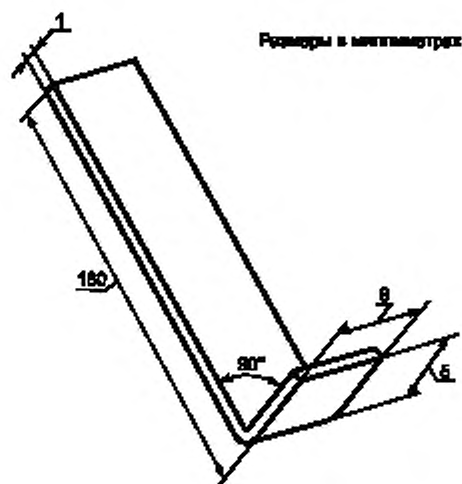
Рисунок 4 — Испытательный крюк
