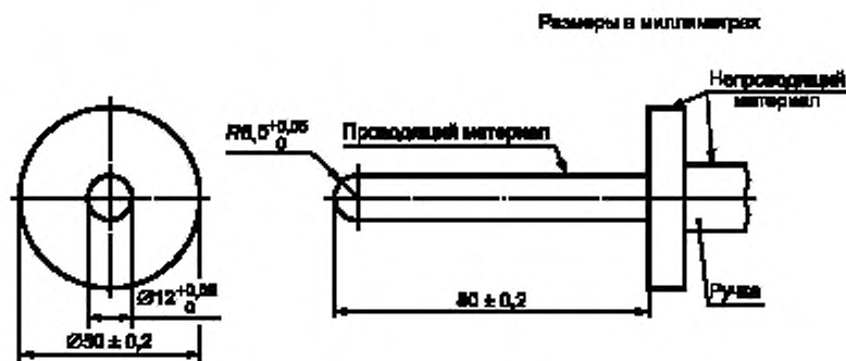
Рисунок В.1 — Испытательный щуп
