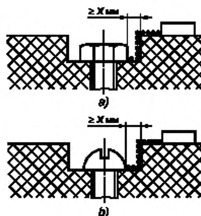
Рисунок E.9 — Малое углубление
