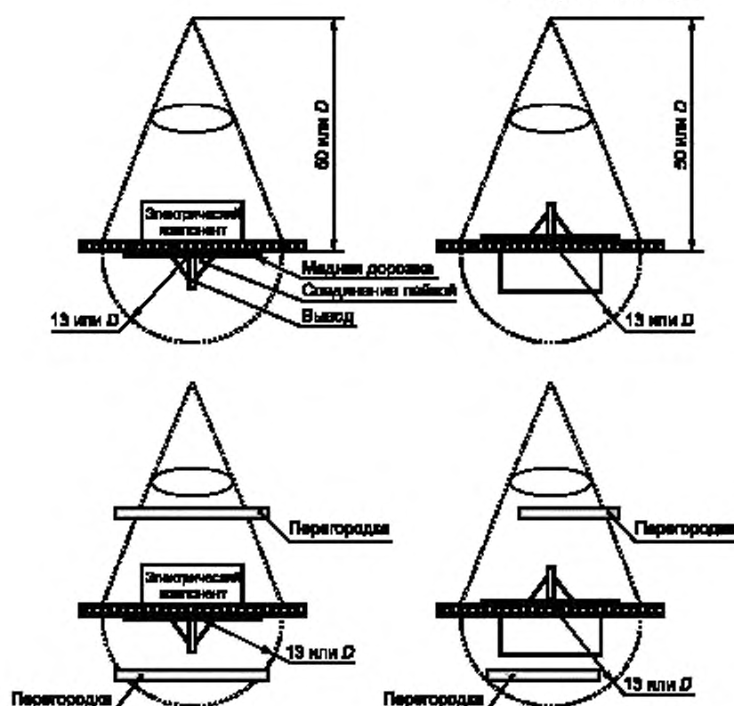
Рисунок 13 — Расстояния от ПОТЕНЦИАЛЬНЫХ ИСТОЧНИКОВ ВОСПЛАМЕНЕНИЯ. Лист 1
