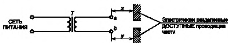
Рисунок 1 — Схема испытательной цепи для условий неисправности
