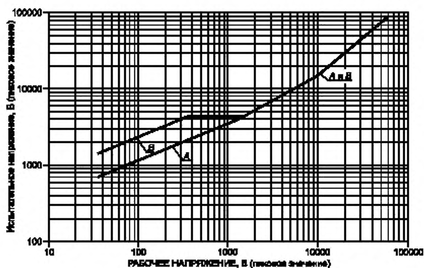
Рисунок 7 — Испытательное напряжение
