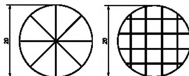
Рисунок 12 — Образцы шарпин для испытаний на взрывоопасность
