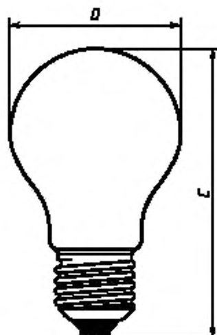
Рисунок 2 — Лампа с резьбовым цоколем Эдисона
