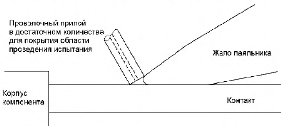
Рисунок 2 — Расположение паяльника
