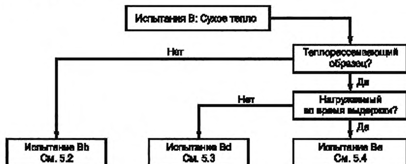
Рисунок 1 — Блок-схема испытаний В: Сухое тепло
