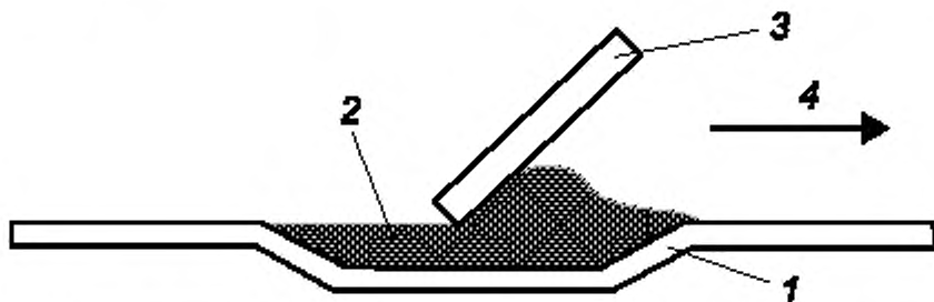
1 — тестовая пластина; 2 — припойная паста; 3 — ракель; 4 — направление движения
