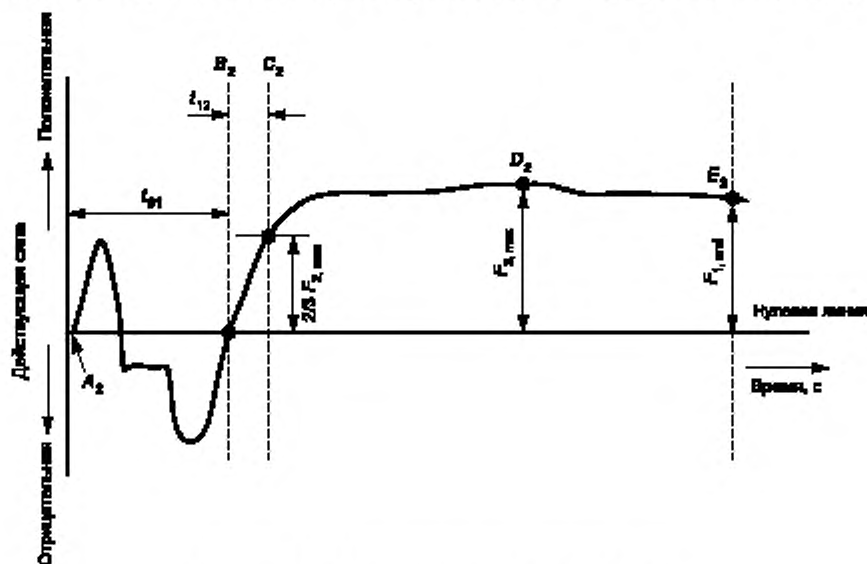
Рисунок Е.3 — Сила смачивания припойной пасты
