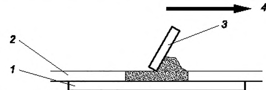
1 — тестовая пластина; 2 — металлическая маска; 3 — ракель; 4 — направление движения ракеля
