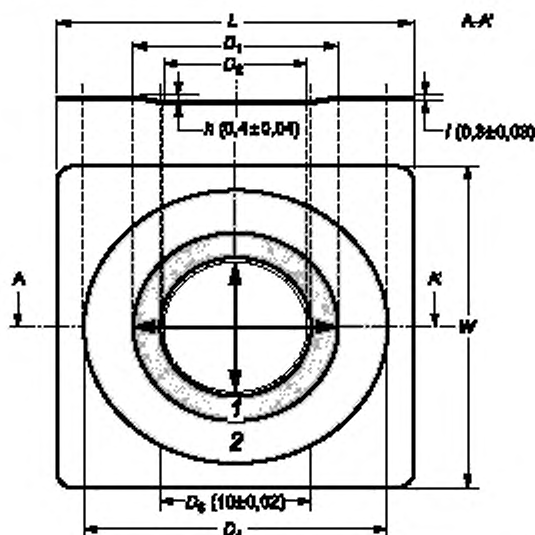
l — граница паяльной маски; 2 — паяльная маска; L, W — внешние размеры; D_1 — внешний диаметр; D_2 — внутренний диаметр; D_3 — внутренний диаметр паяльной маски; D_4 — внешний диаметр паяльной маски; h — глубина пластины; l — толщина
