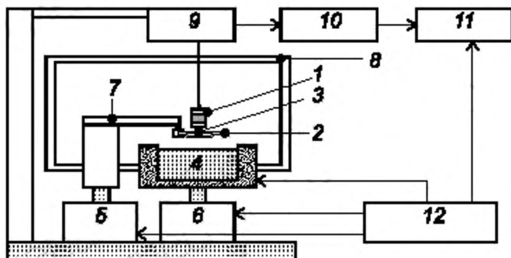
1 — образец; 2 — испытательный стенд в виде пластины; 3 — припойная паста; 4 — нагревательная ванна; 5 — лифт для пластины; 6 — лифт для нагревательной ванны; 7 — зажимное устройство для пластины; 8 — корпус; 9 — датчик; 10 — преобразователь сигнала; 11 — записывающее устройство; 12 — контроллер
