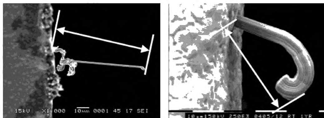
Рисунок А.1 — Определение длины усов
