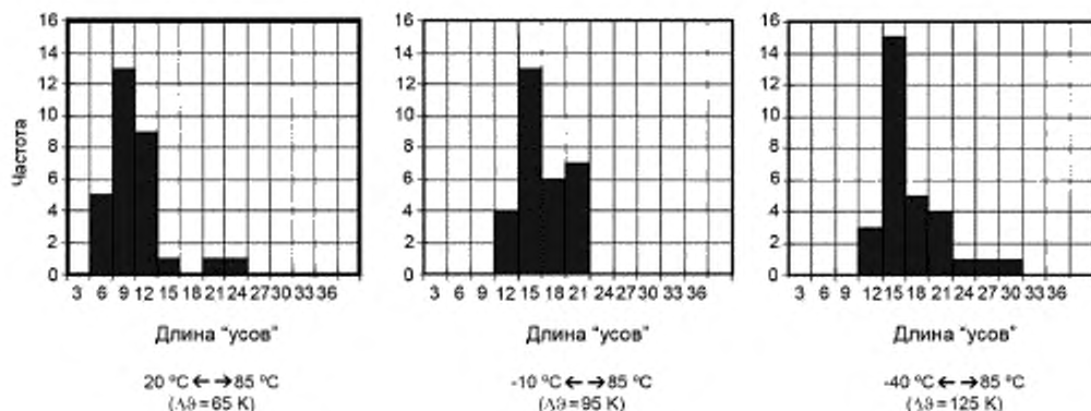
Рисунок Н.1 — Распределения длины усов, выросших на основном материале
