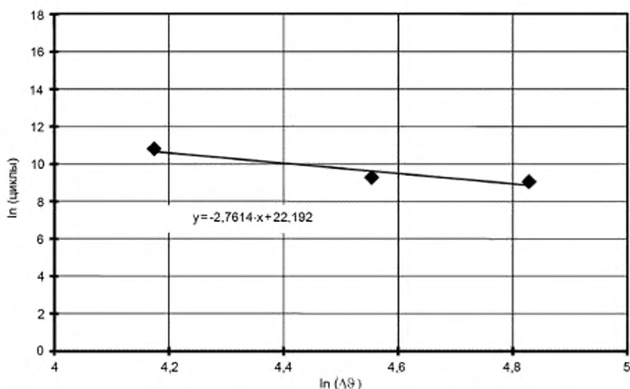
Рисунок Н.3 — Зависимость между \Delta\theta и числом циклов для роста усов на основном материале, сплав 42
