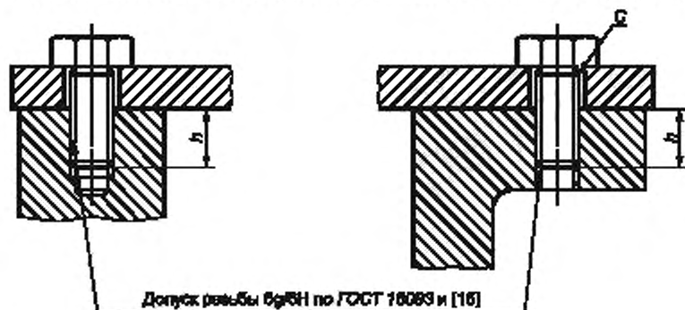
Рисунок 1 — Допуски и зазор для резьбовых крепежных деталей
