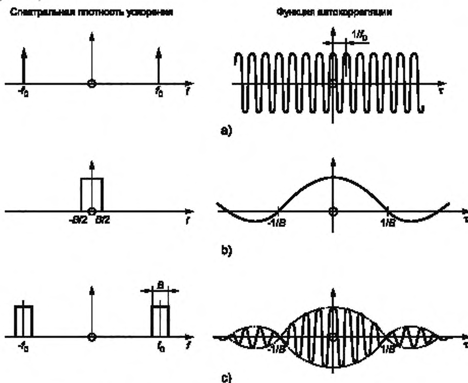
Рисунок 3 — Функции автокорреляции разных сигналов 1)
