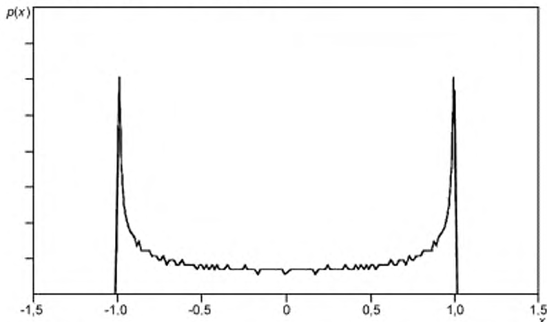
Рисунок 1 — Плотность распределения вероятностей для гармонического сигнала
