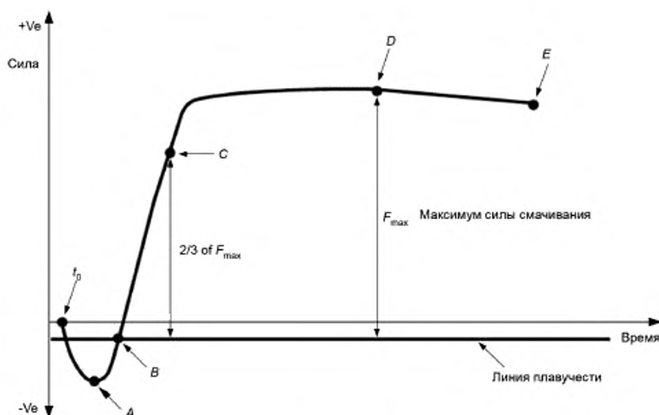
Рисунок 2 — Условия смачивания
