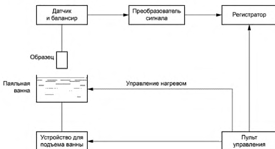
Рисунок 1 — Блок-схема для испытания
